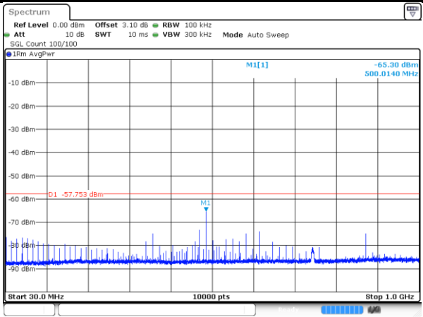
4955-10MHz-802.11n-2-a
