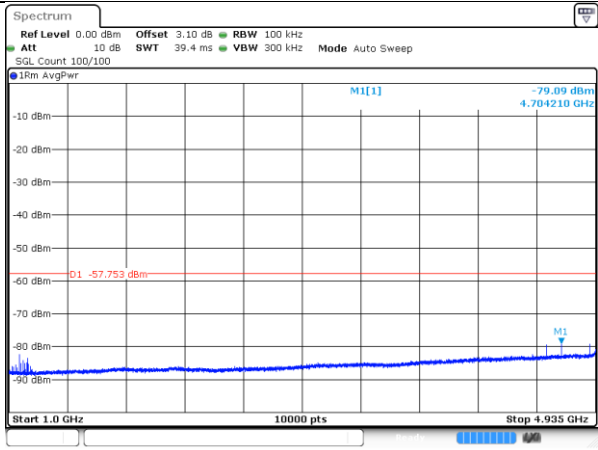
4955-10MHz-802.11n-2-a
