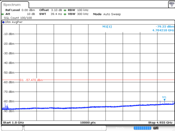
4950-10MHz-802.11n-2-as
