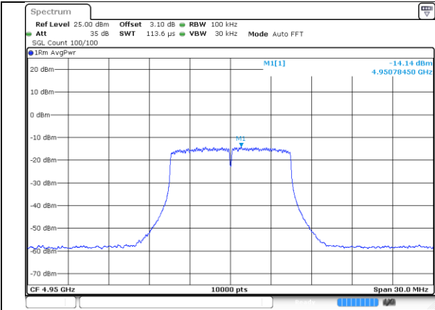
4950-10MHz-802.11n-1-a
