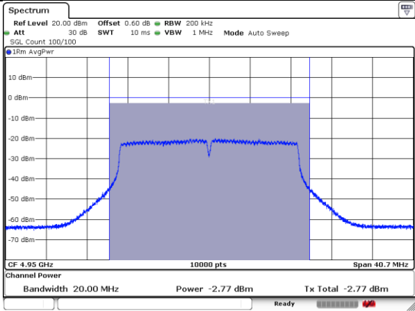
4950MHz-20MHz-802.11ac-2-b
