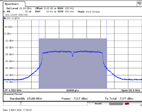
4955MHz-10MHz-802.11ac-2-b
