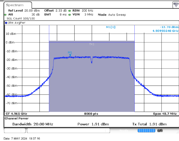
4965MHz-20MHz-802.11ac-1-15-b
