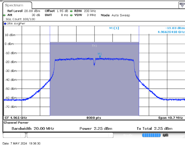
4965MHz-20MHz-802.11ac-1-15-a
