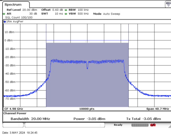
4980MHz-20MHz-802.11ac-2-a
