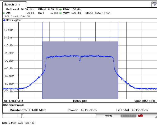
4955MHz-10MHz-802.11ac-2-a
