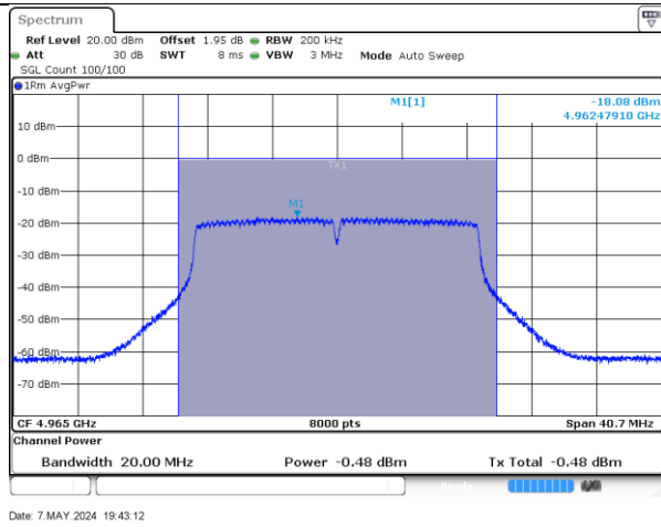
4965MHz-20MHz-802.11ac-2-a
