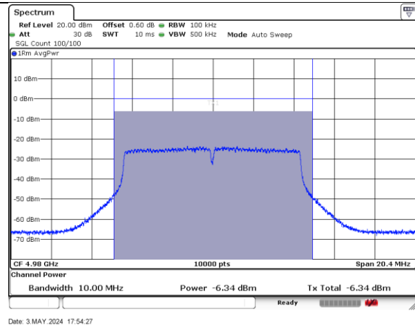
4980MHz-10MHz-802.11ac-2-b
