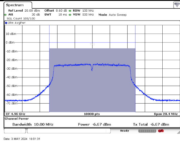
4950MHz-10MHz-802.11ac-2-b
