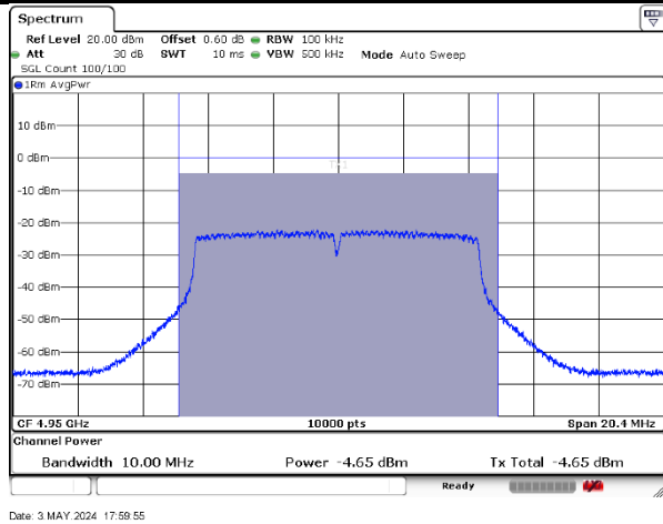
4950MHz-10MHz-802.11ac-2-a
