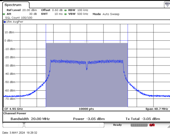
4950MHz-20MHz-802.11ac-2-a
