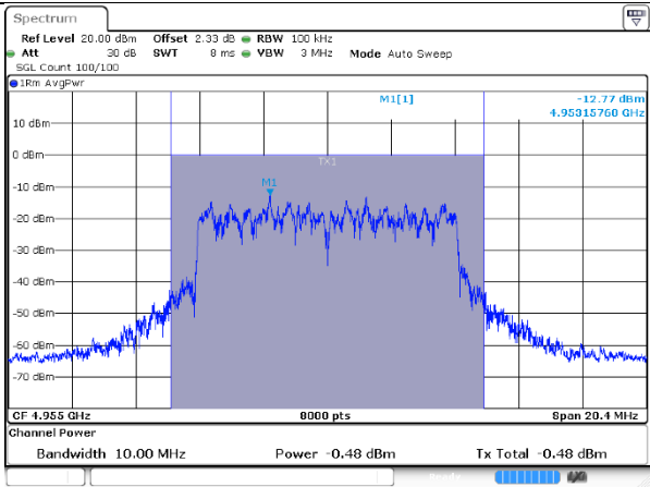
4950MHz-10MHz-802.11a-2-b
