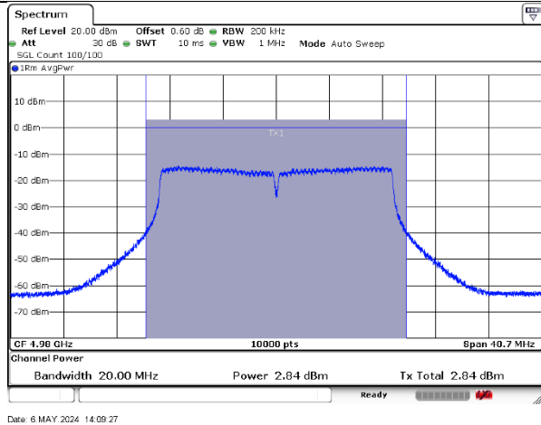
4980MHz-20MHz-802.11ac-1-a
