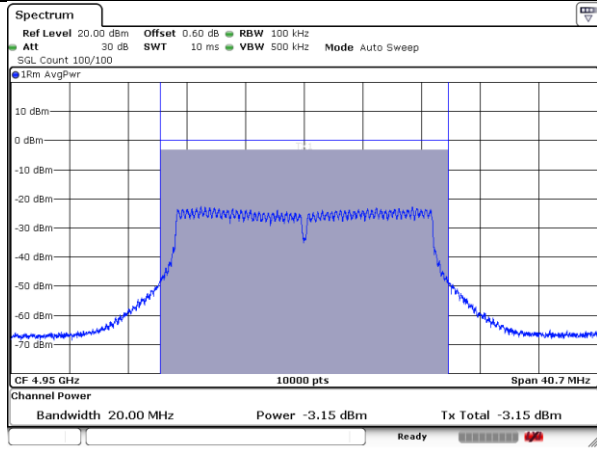
4950MHz-20MHz-802.11n-2-a
