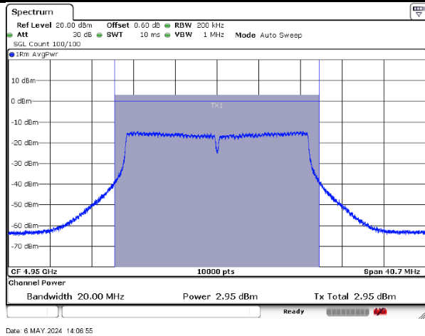
4950MHz-20MHz-802.11ac-1-a
