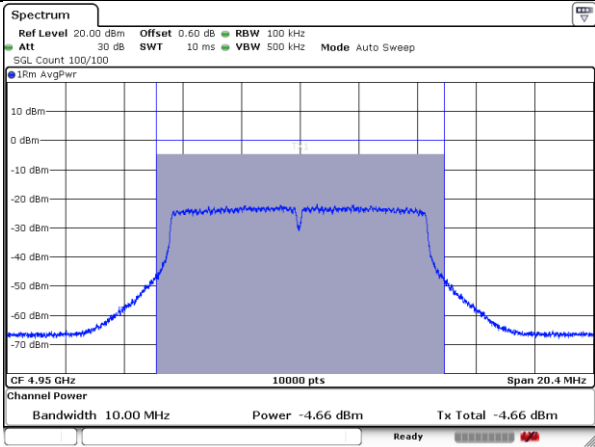
4950MHz-10MHz-802.11n-2-a
