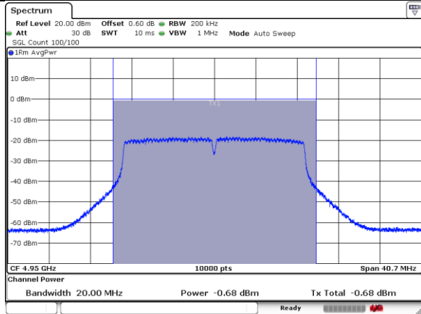
4950MHz-20MHz-802.11n-2-a
