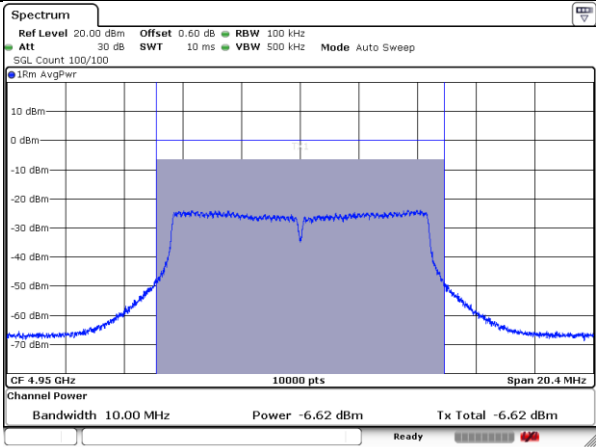
4950MHz-10MHz-802.11ac-2-a
