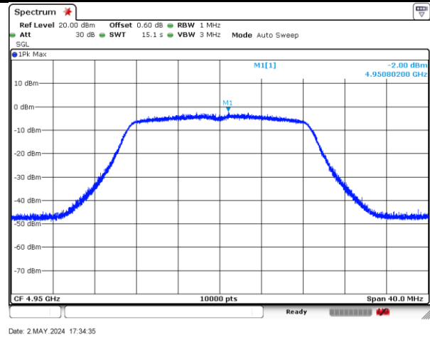
4950-20MHz-802.11n-2-b
