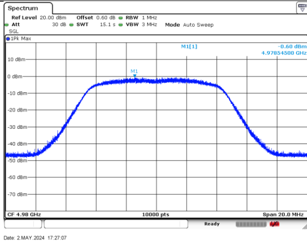
4980-10MHz-802.11n-2-a
