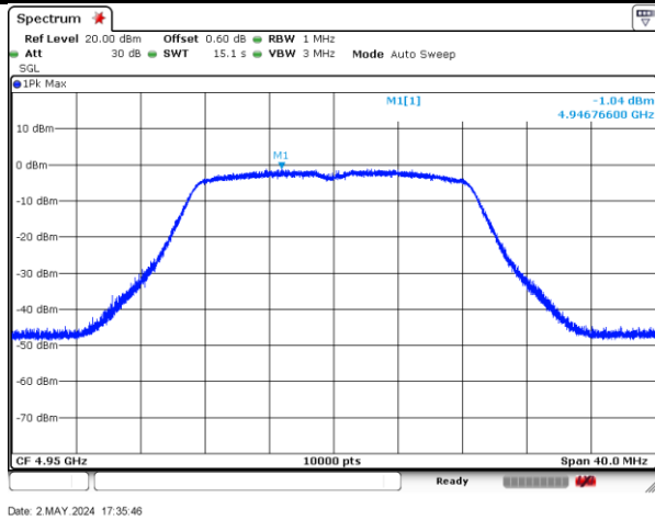
4950-20MHz-802.11n-2-a
