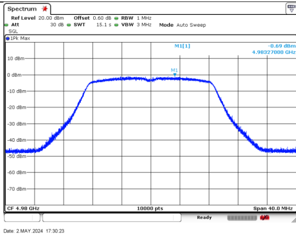
4980-20MHz-802.11n-2-a
