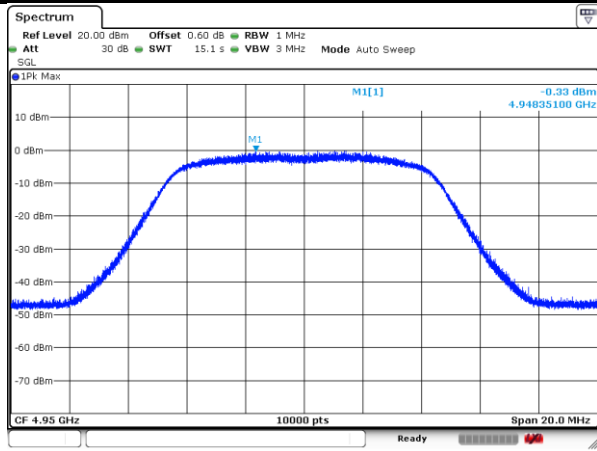
4950-10MHz-802.11n-2-a
