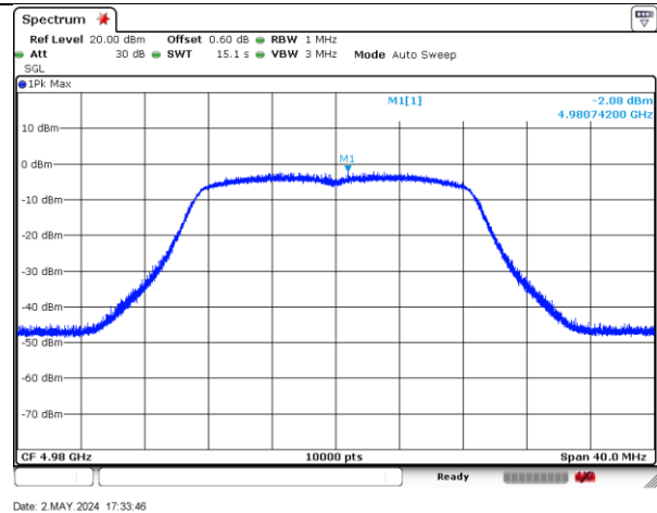
4980-20MHz-802.11n-2-b
