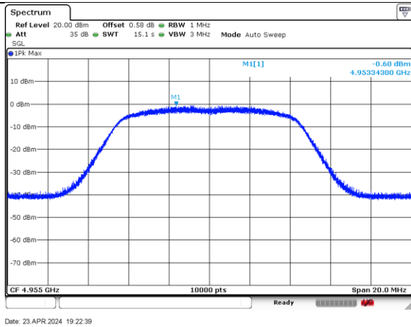
4955-10MHz-802.11n-2-a
