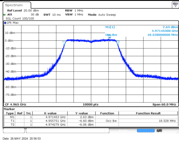
4965MHz-20MHz-802.11n-Radio_2
