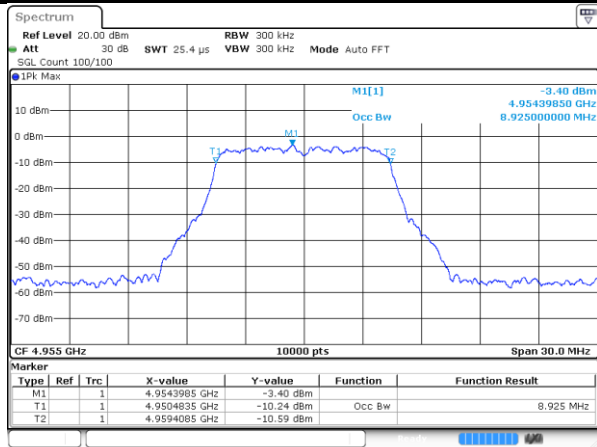
4955MHz-10MHz-802.11n-Radio_1
