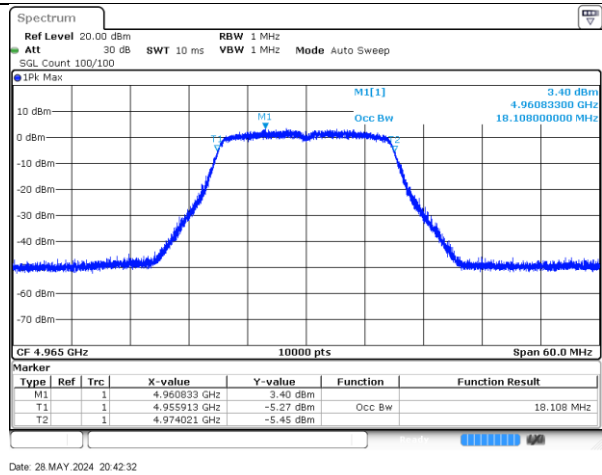
4965MHz-20MHz-802.11ac-Radio_1
