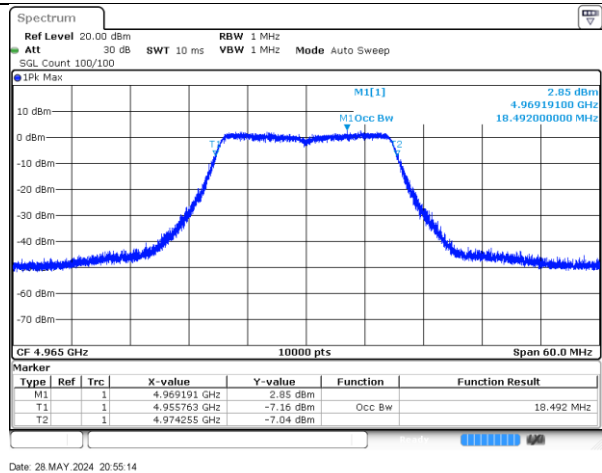
4965MHz-20MHz-802.11ac-Radio_2
