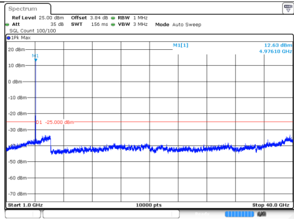
4980-10MHz-802.11a-1-a
