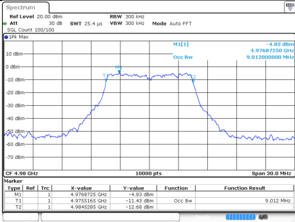
4980MHz-10MHz-802.11ac-Radio_2
