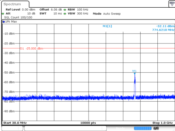
4980-10MHz-802.11a-2-a
