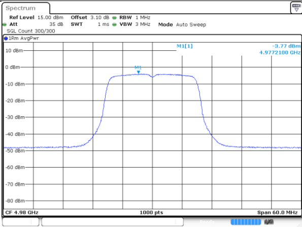
4980-20MHz-802.11n-1-a
