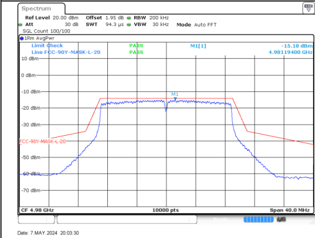
4980MHz-20MHz-802.11ac-Radio_1
