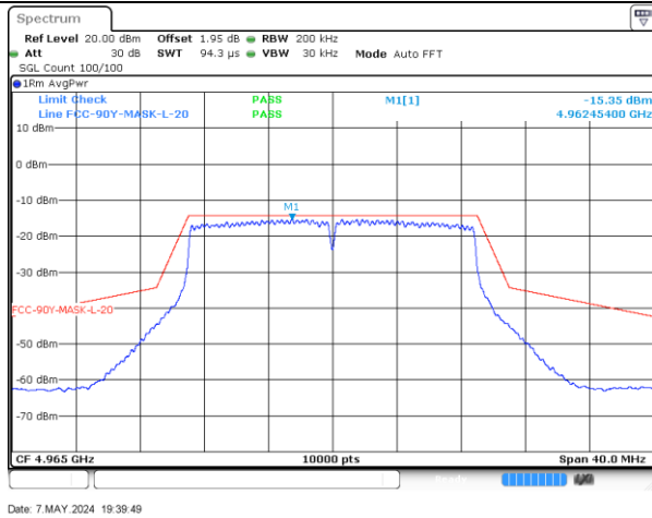
4965MHz-20MHz-802.11n-Radio_1
