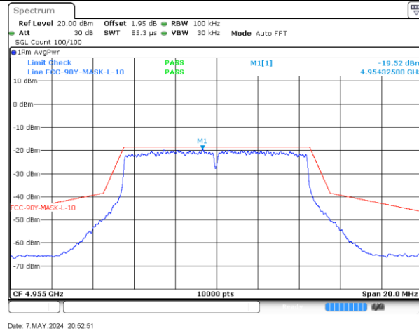
4955MHz-10MHz-802.11ac-Radio_1
