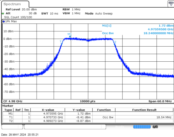
4980MHz-20MHz-802.11ac-Radio_2
