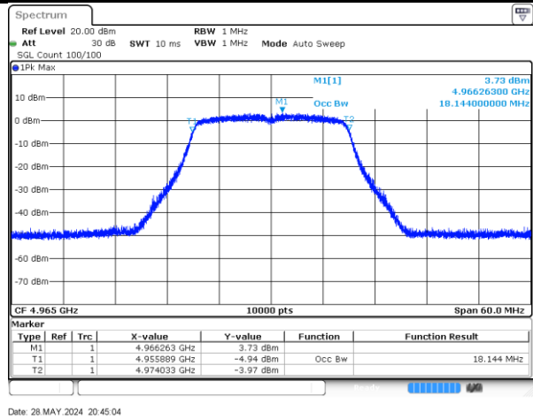
4965MHz-20MHz-802.11n-Radio_1
