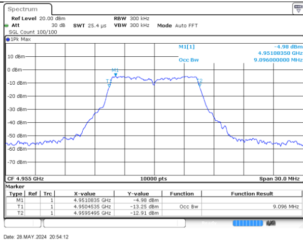
4955MHz-10MHz-802.11ac-Radio_2
