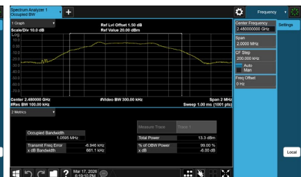
CH39
