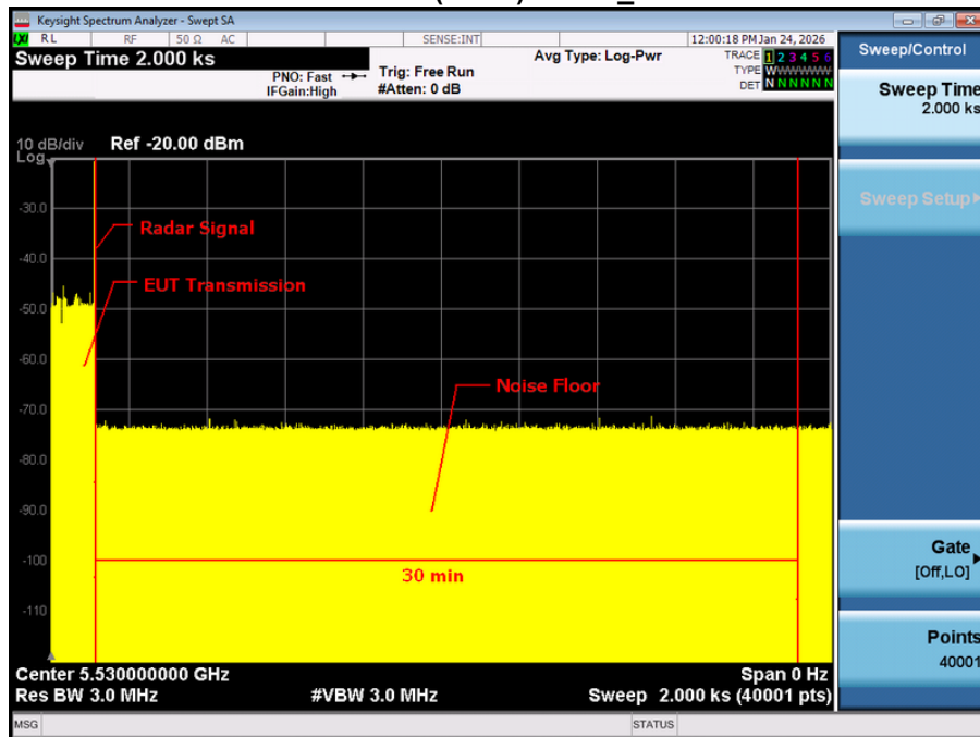
IEEE 802.11ax(HE80) Mode _5530MHz
