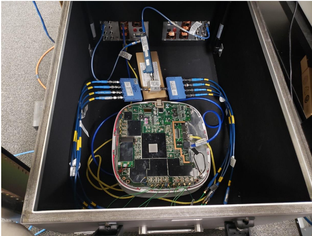
EUT Photo
