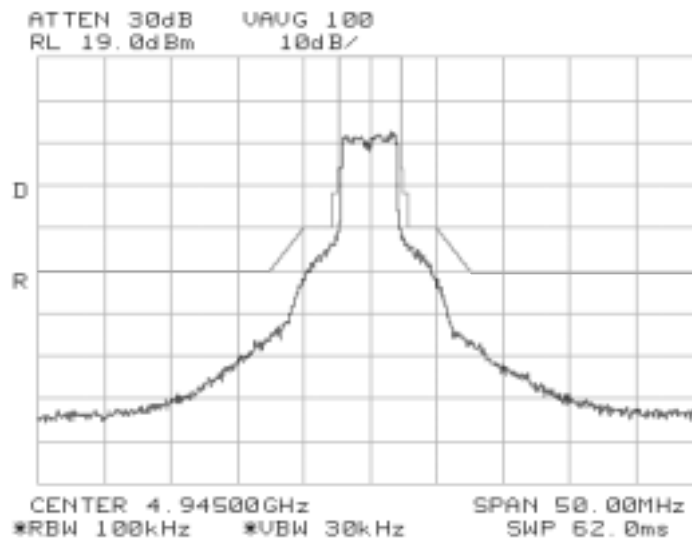
5MHz (4945 MHz)
