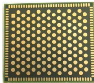
Fig. 2. FANW module bottom view
