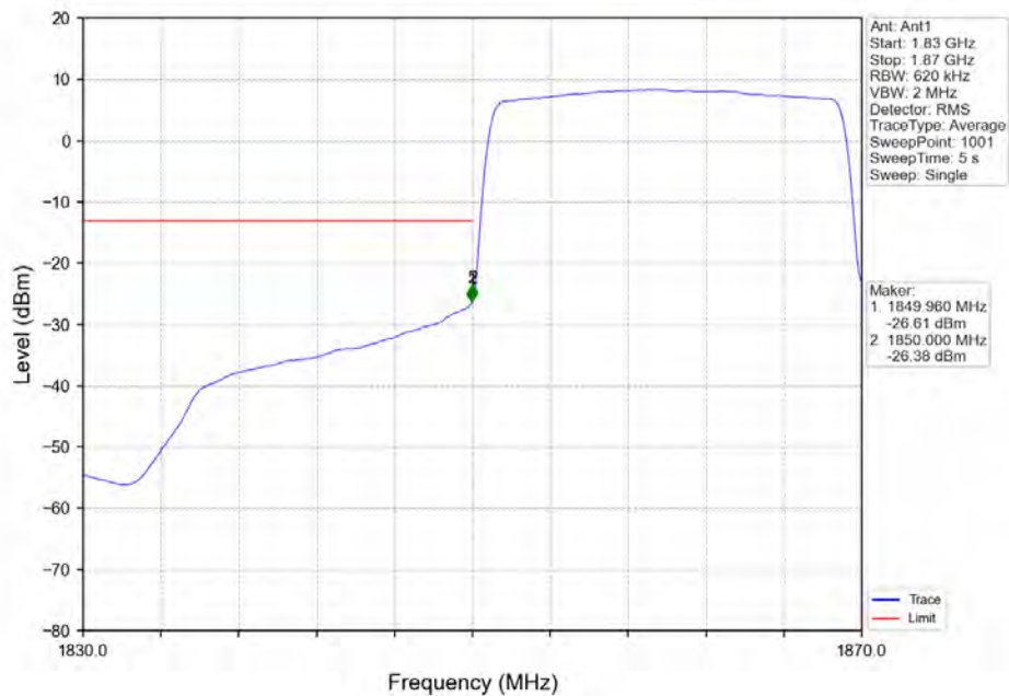
Band_25_20MHz_16QAM_LCH_1860MHz_RB_100_0_NTNV
