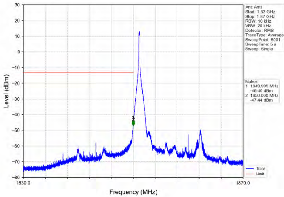
Band_25_20MHz_QPSK_LCH_1860MHz_RB_1_0_NTNV
