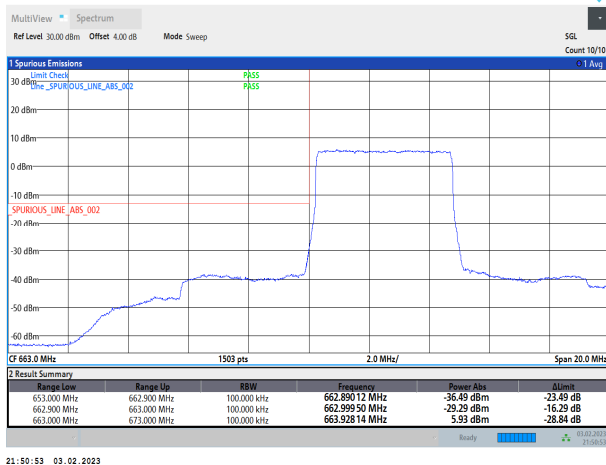
Band71-5MHz-QPSK-133147-25RB#0
