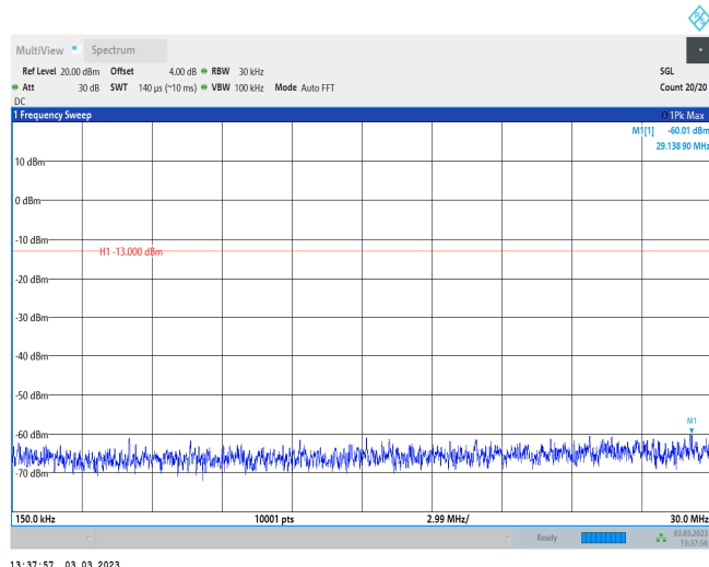
GSM850-128-0.15~30MHz
