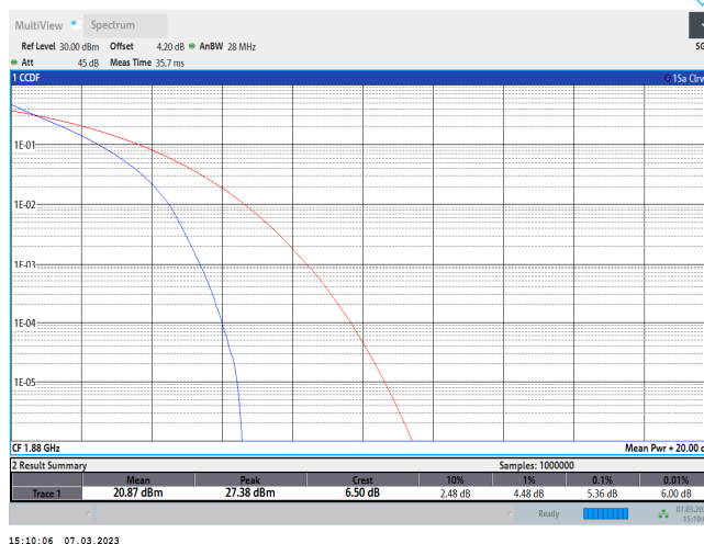
Band2-20MHz-QPSK-18900-100RB#0
