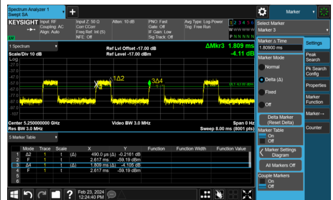
802.11be-EHT160 (5250MHz)
