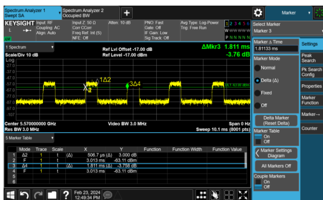
802.11be-EHT160 (5570MHz)
