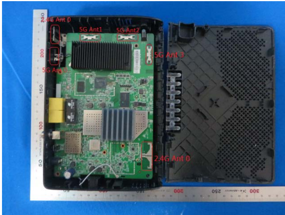
(1) EUT Photo (WCB6200Q)
