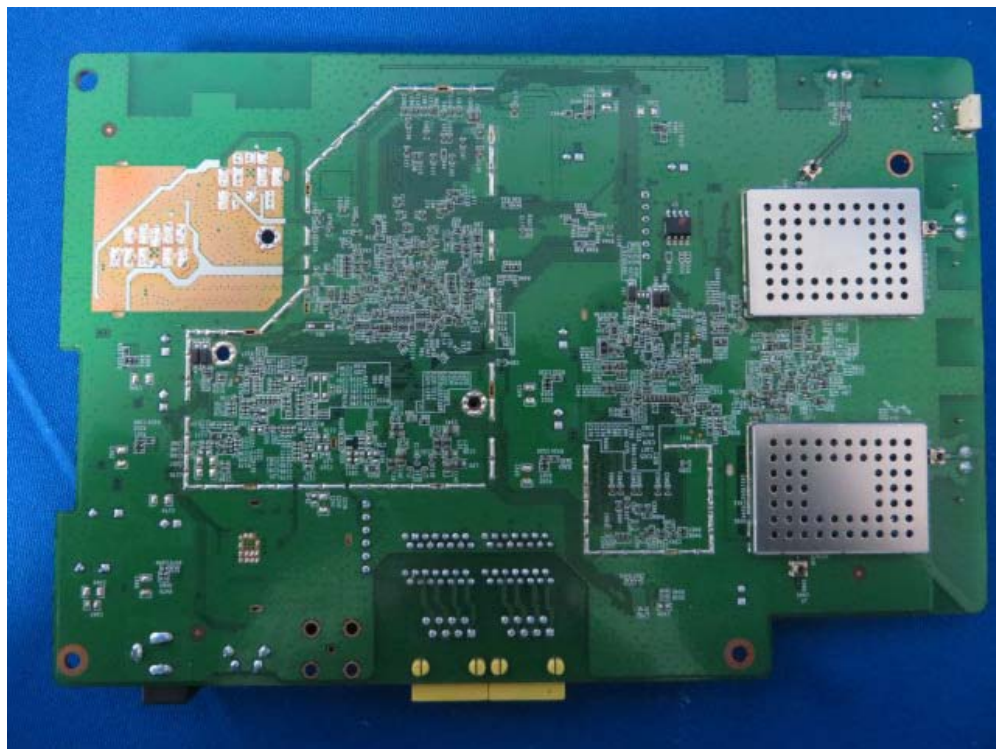
(30) EUT Photo (WEB6000Q)
