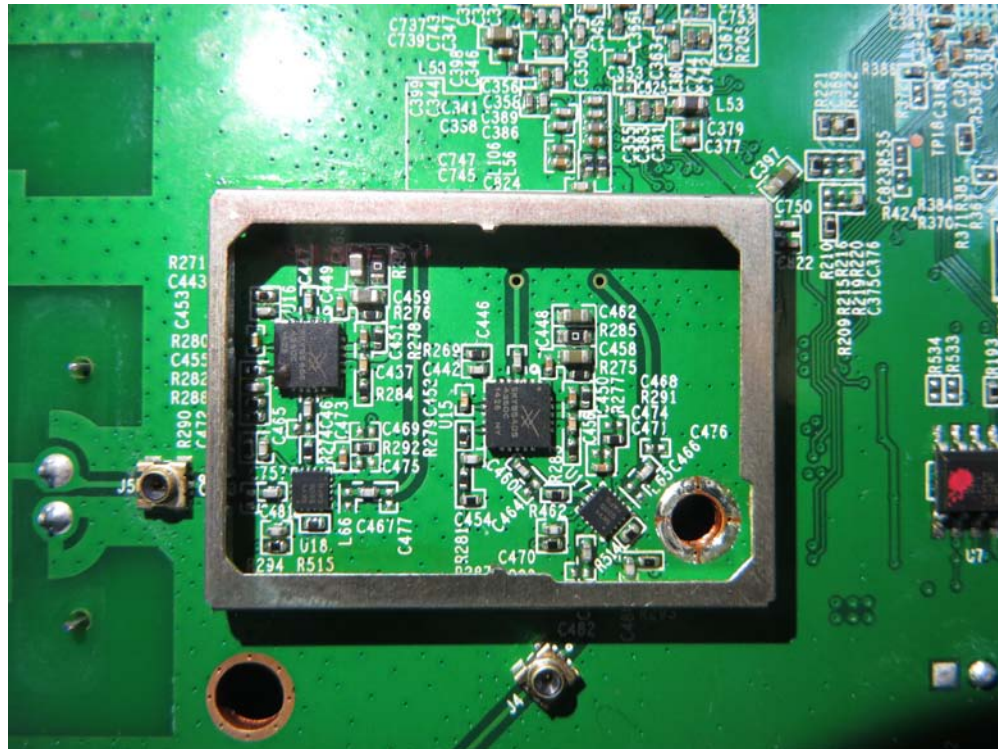
(35) EUT Photo (WEB6000Q)
