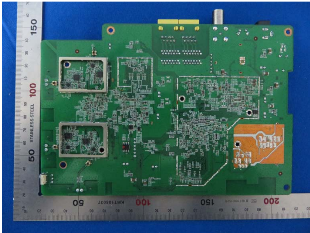
(24) EUT Photo (WCB6000Q)
