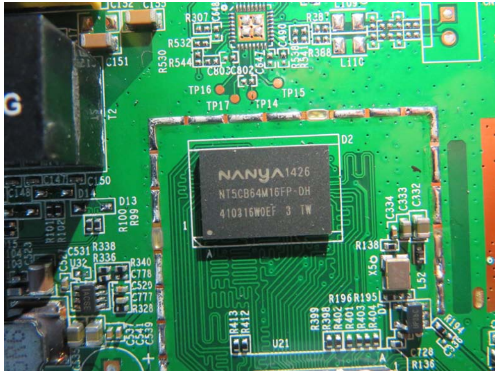
(7) EUT Photo (WCB6200Q)
