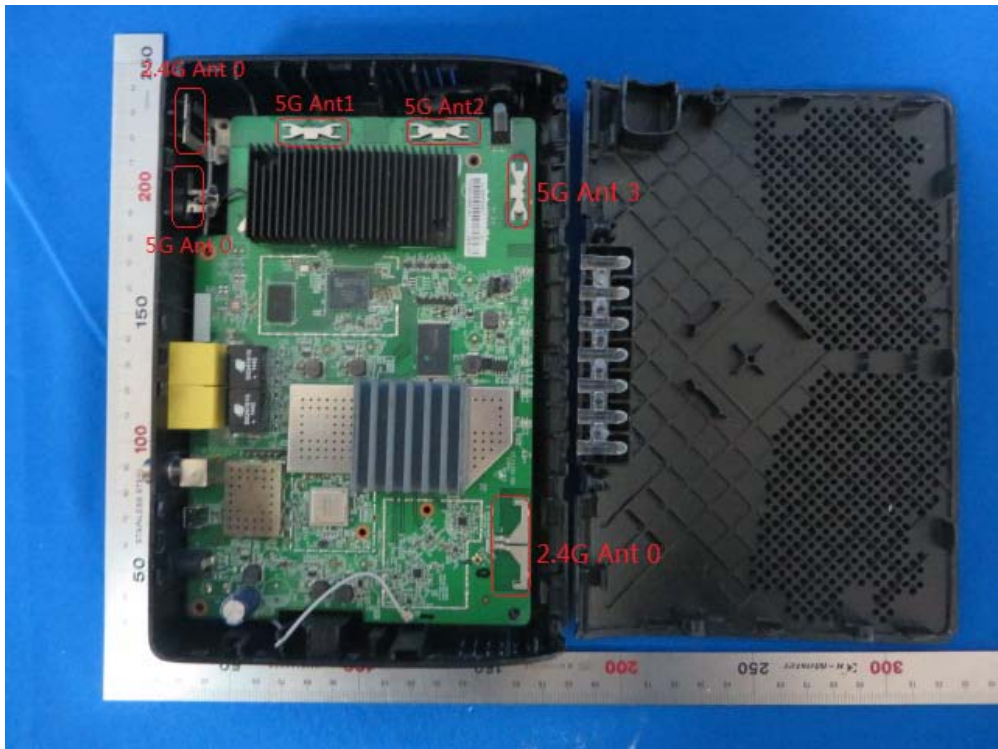
(14) EUT Photo (WCB6000Q)
