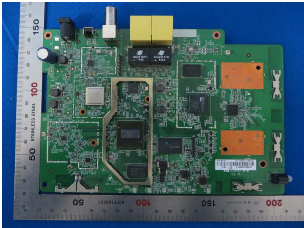
(18) EUT Photo (WCB6000Q)
