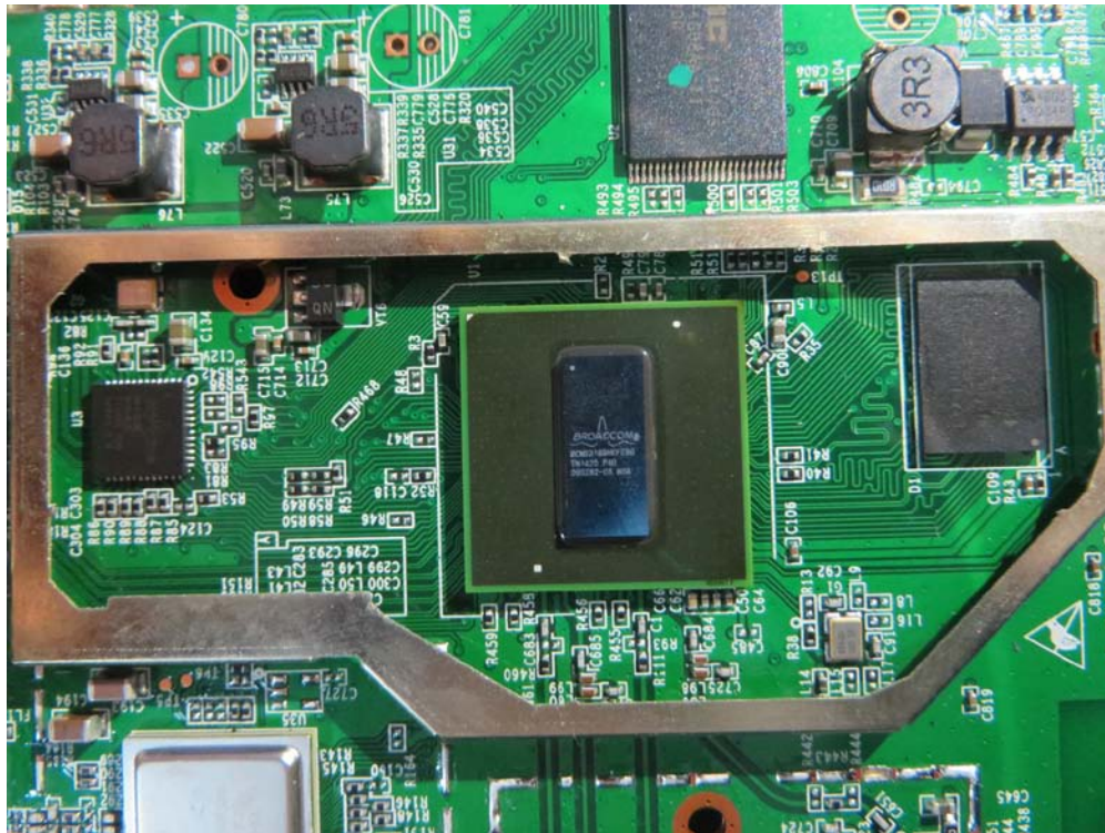
(9) EUT Photo (WCB6200Q)
