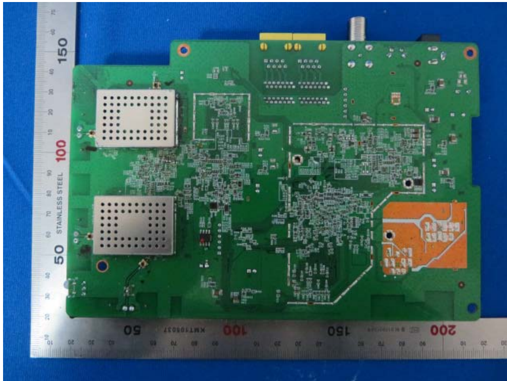
(17) EUT Photo (WCB6000Q)
