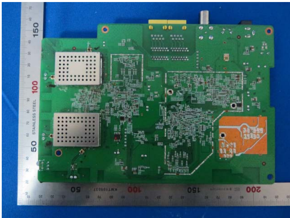
(4) EUT Photo (WCB6200Q)
