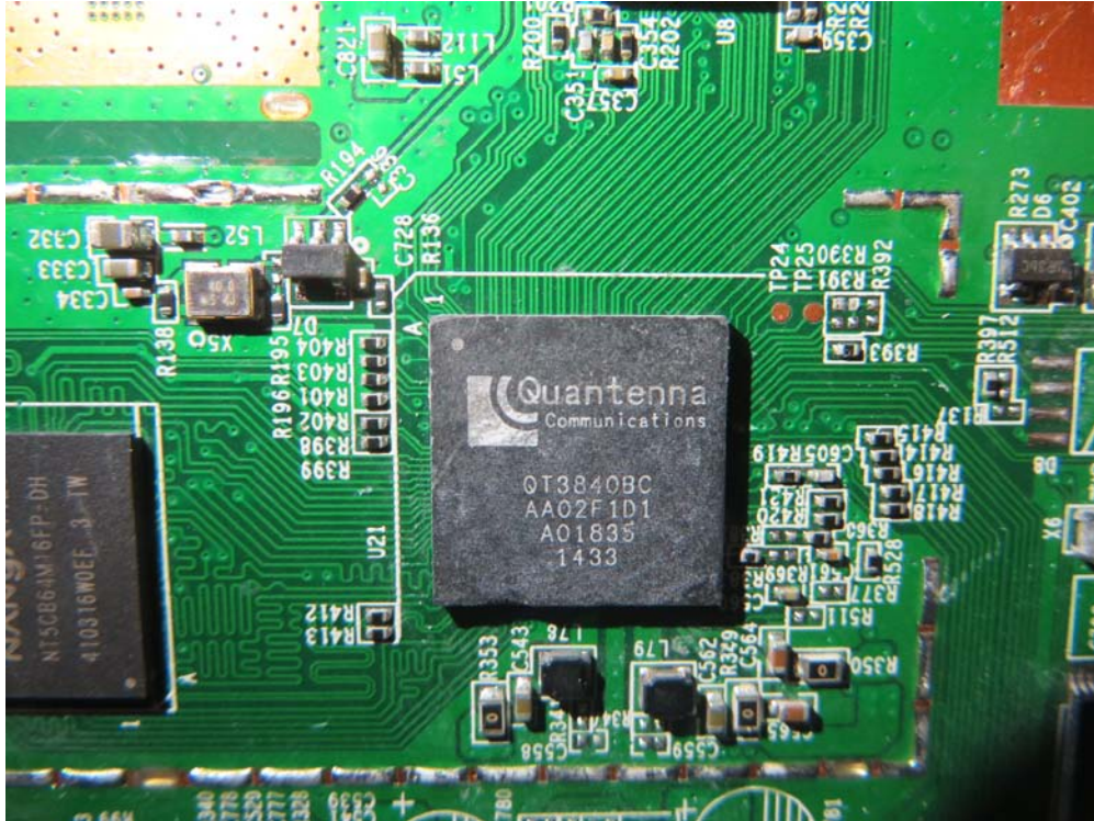
(32) EUT Photo (WEB6000Q)
