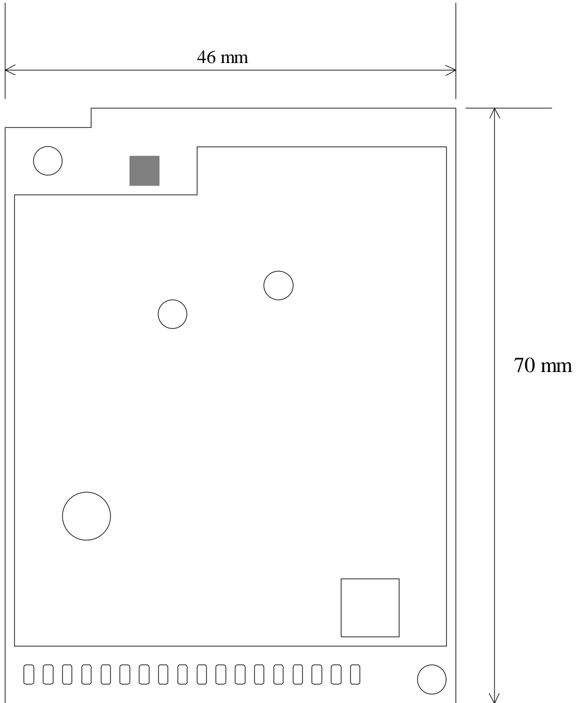
900 MHz RF Module Dimensions
