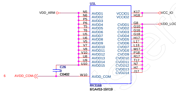
RK3168_L
