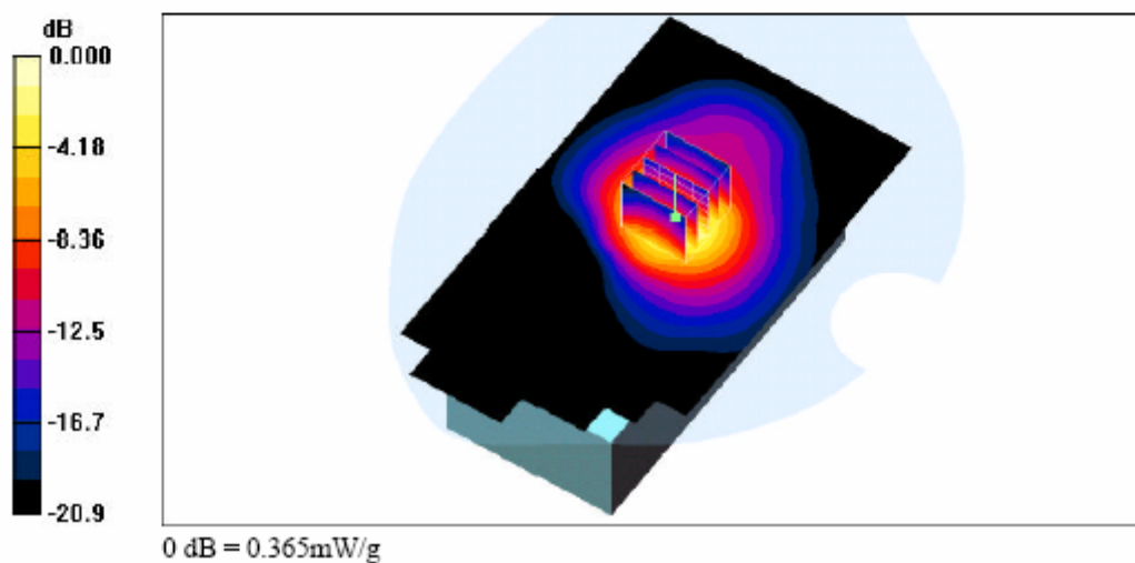
IEEE 802.11b Body SAR _CH 1
