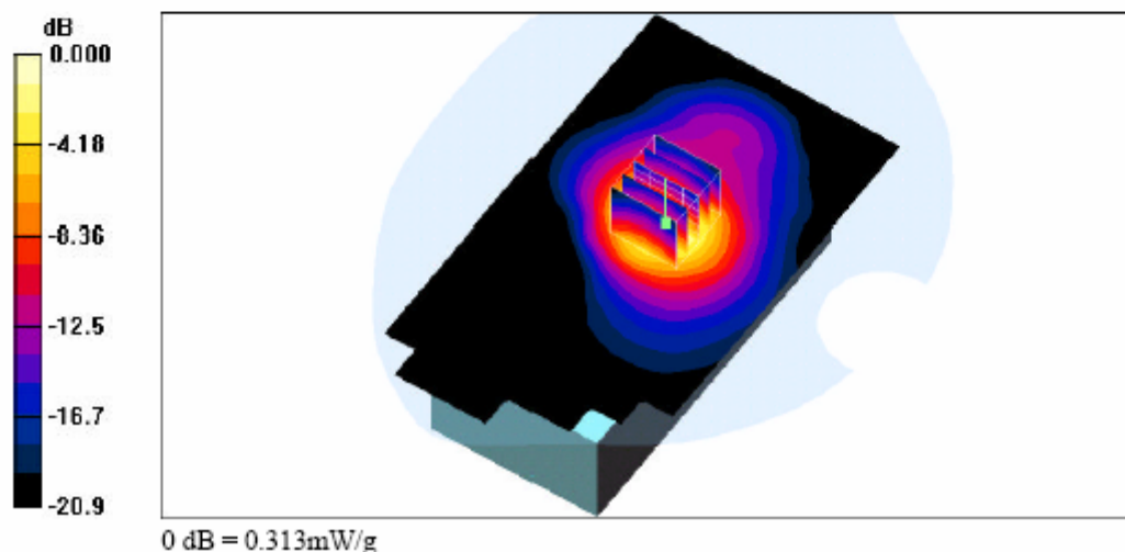
IEEE 802.11b Body SAR _CH 11
