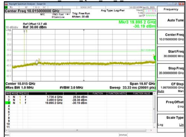
Band4 20MHz QPSK RB1 0 CH20300
