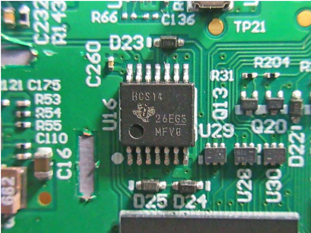
(40) EUT Photo
