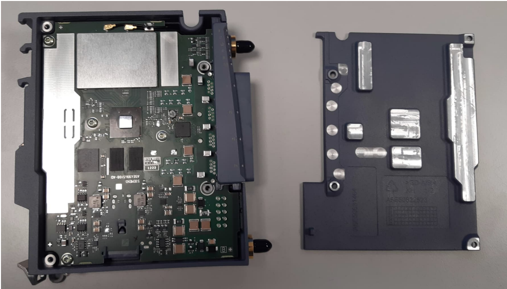
PCB A-Side
