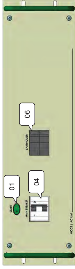
MCCB AC Mains M208 / B240 (Front View)
