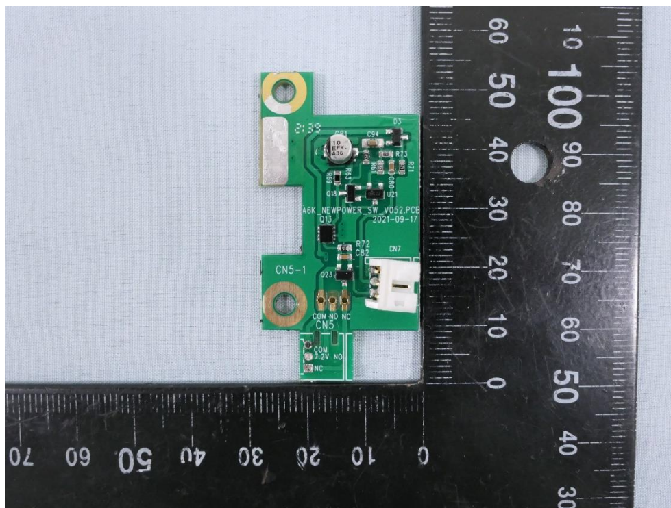
(20) EUT Photo (TX)
