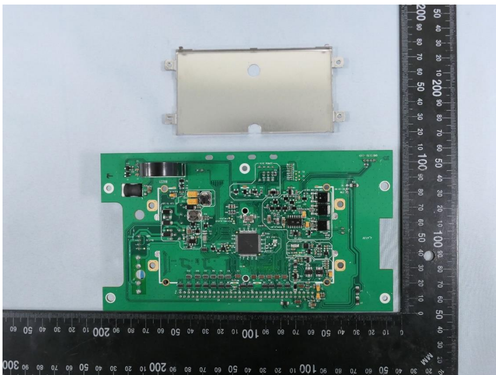
(14) EUT Photo (TX)
