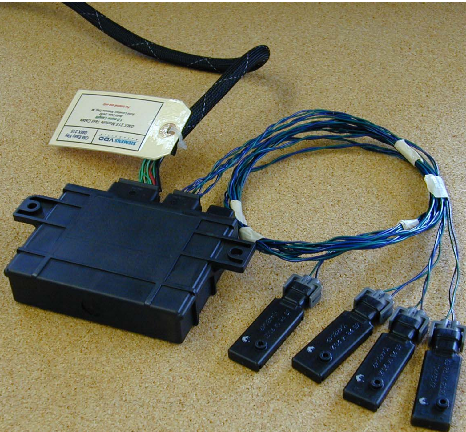
DUT (bottom)
