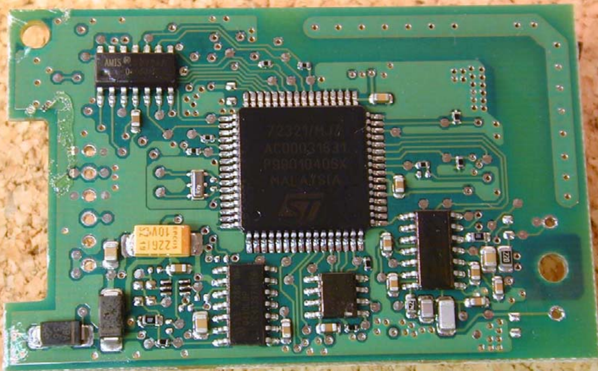
PCB Bottom (5WY7229)
