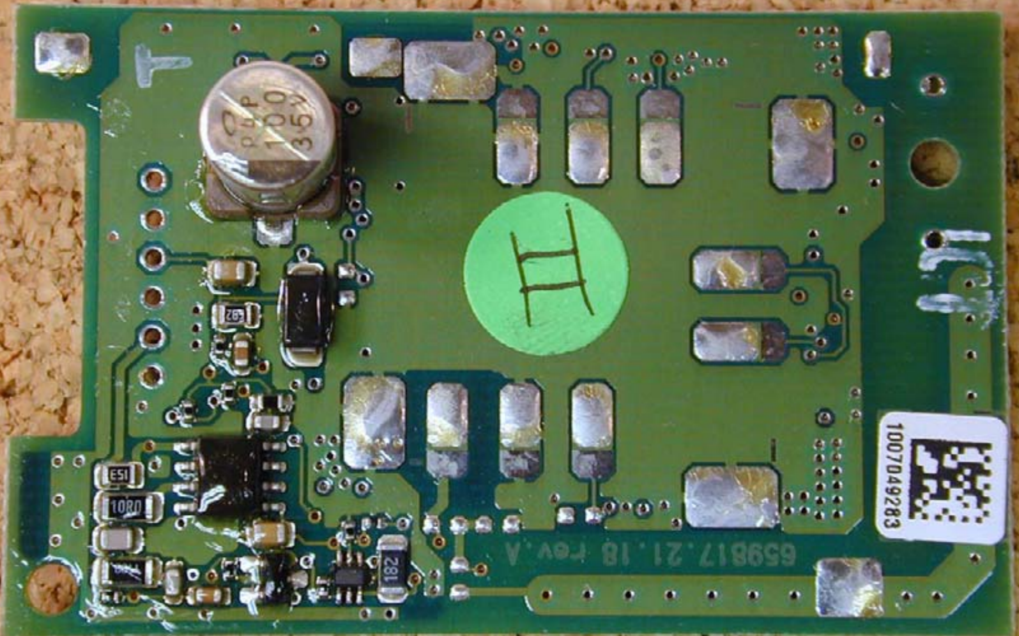
PCB Top (5WY7229)
