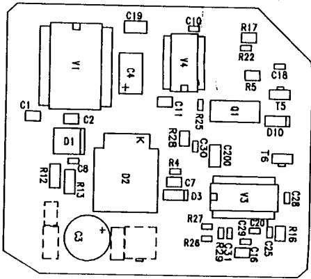
TOP SIDE
