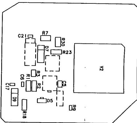
BOTTOM SIDE
