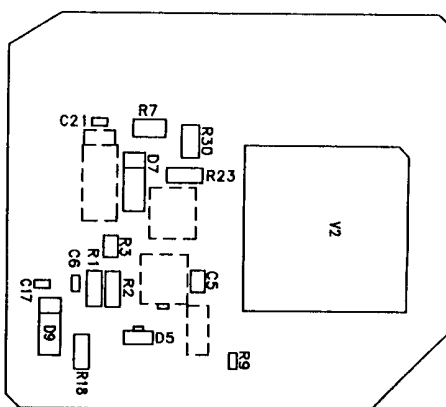
BOTTOM SIDE
