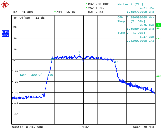
802.11n20_2412MHz_Chain 0
