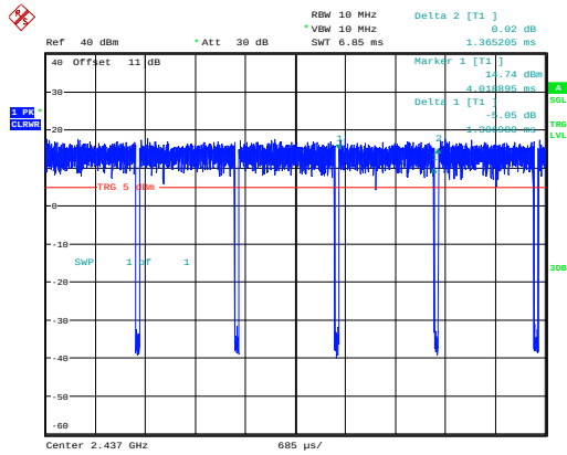
802.11n20_2437MHz_Chain 0
