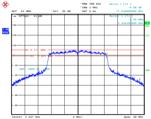
802.11n20_2437MHz_Chain 0
