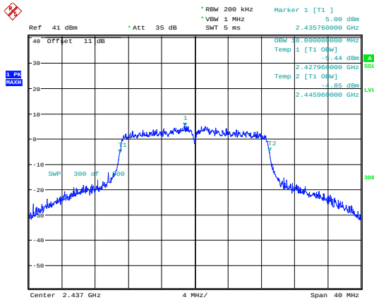
802.11n20_2437MHz_Chain 0
