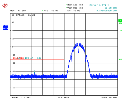
802.11b_2412MHz_Chain 1
