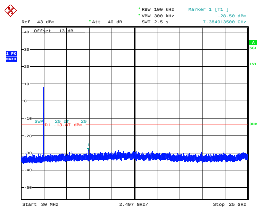
802.11b_2462MHz_Chain 0
