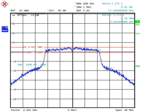
802.11n20_2462MHz_Chain 0
