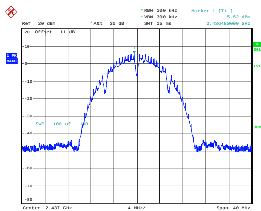
802.11b_2437MHz_Chain 1
