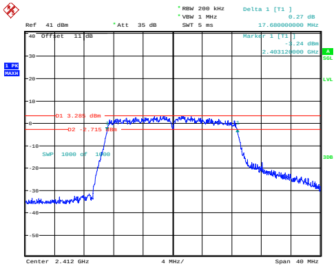
802.11n20_2412MHz_Chain 0
