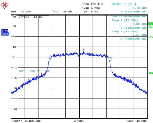
802.11n20_2462MHz_Chain 0
