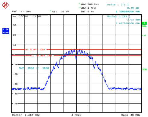
802.11b_2412MHz_Chain 0
