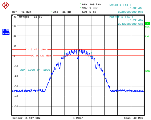
802.11b_2437MHz_Chain 0
