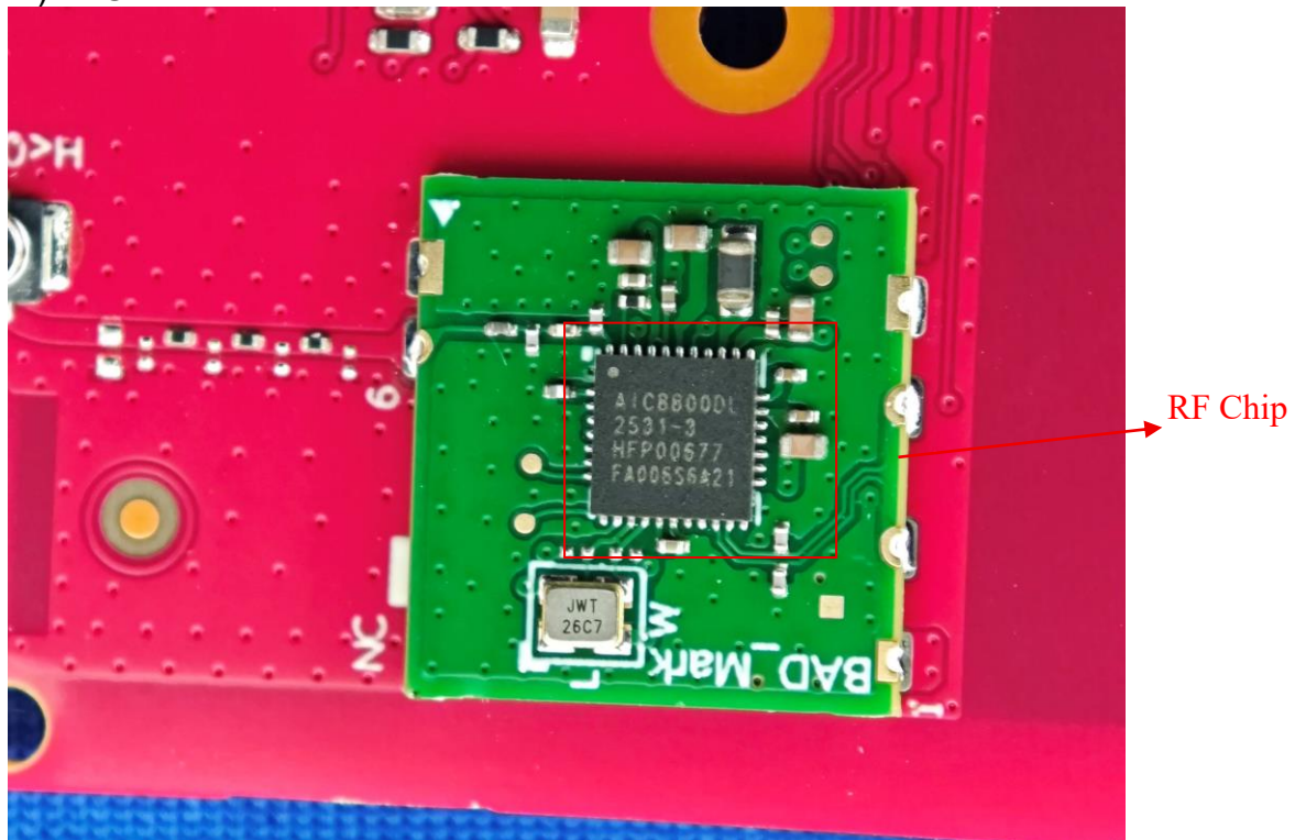
7) EUT Photo
