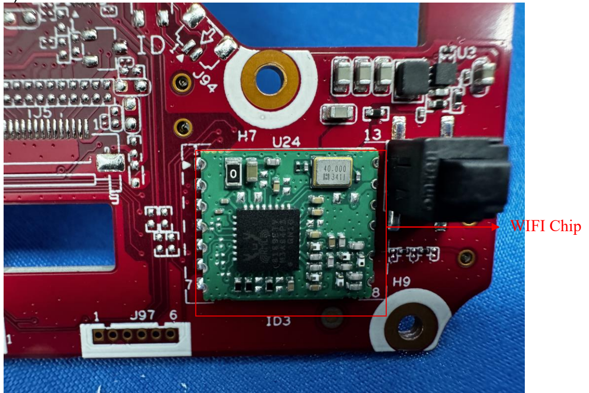
8) EUT Photo
