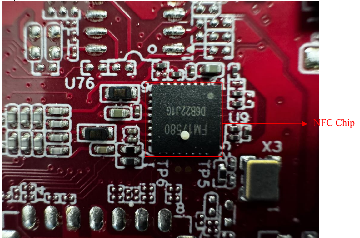
16) EUT Photo
