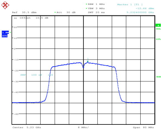
802.11ac40_5230MHz_Chain 0
