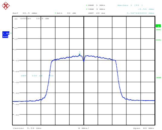
802.11n40_5590MHz_Chain 0
