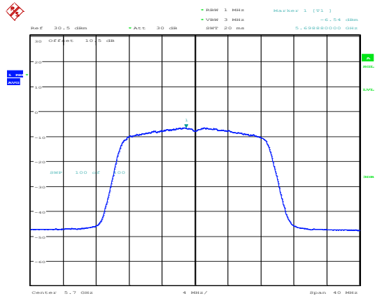
802.11ac20_5700MHz_Chain 1
