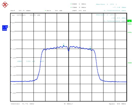
802.11ac40_5710MHz_Chain 1
