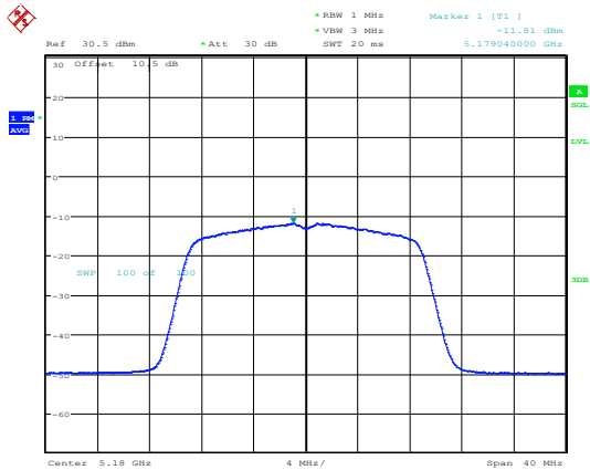
802.11n20_5180MHz_Chain 1
