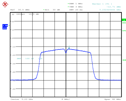
802.11ac40_5230MHz_Chain 1
