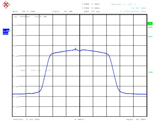
802.11ac20_5260MHz_Chain 0
