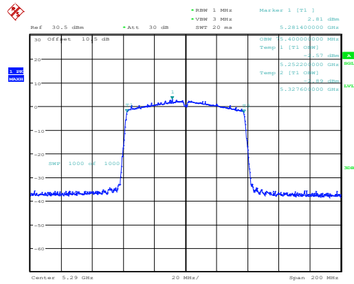
802.11ac80_5290MHz_Chain 0
