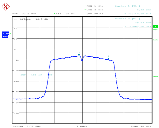
802.11n40_5710MHz_Chain 1
