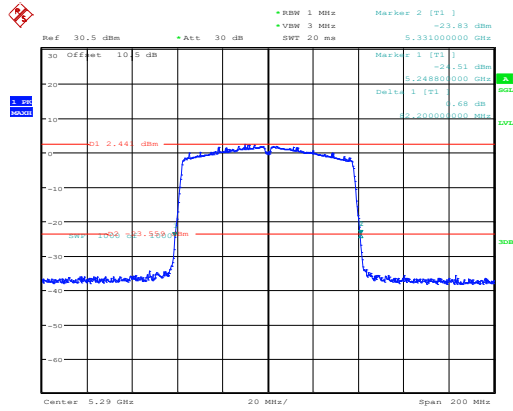
802.11ac80_5290MHz_Chain 0
