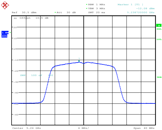
802.11ac20_5240MHz_Chain 0
