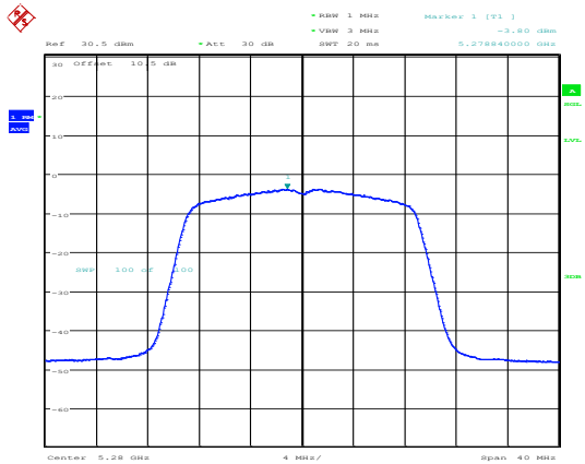
802.11ac20_5280MHz_Chain 0
