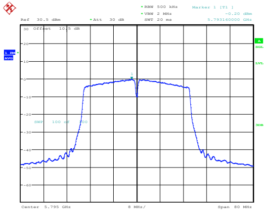
802.11n40_5795MHz_Chain 1
