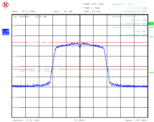
802.11n40_5310MHz_Chain 0
