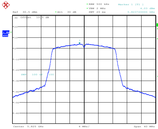
802.11ac20_5825MHz_Chain 1
