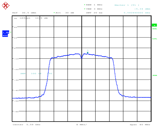
802.11n40_5590MHz_Chain 1
