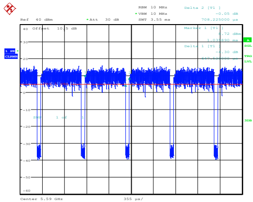
802.11n40_5590MHz_Chain 0
