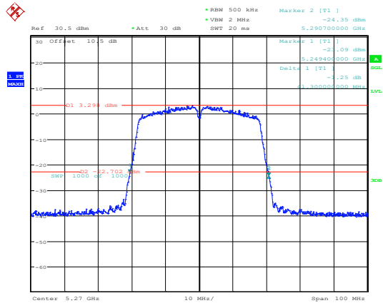
802.11n40_5270MHz_Chain 0
