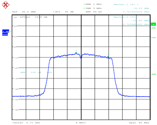
802.11n40_5710MHz_Chain 0
