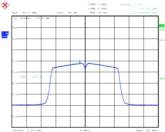
802.11ac40_5190MHz_Chain 0
