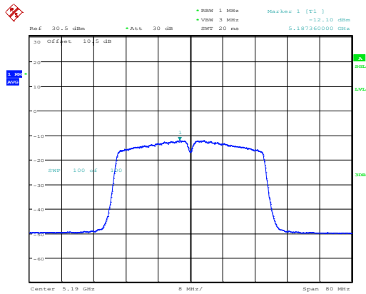
802.11ac40_5190MHz_Chain 1
