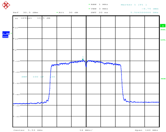
802.11ac80_5530MHz_Chain 1
