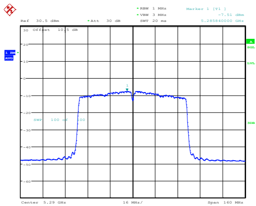
802.11ac80_5290MHz_Chain 0
