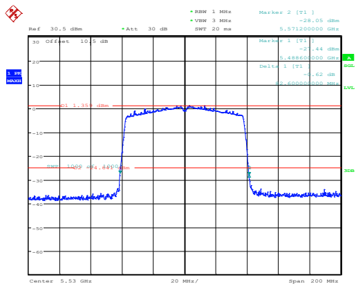
802.11ac80_5530MHz_Chain 0
