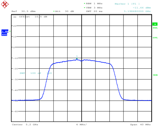
802.11ac20_5200MHz_Chain 1
