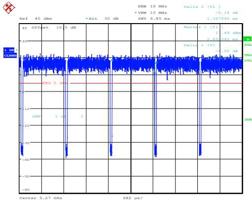
802.11n40_5270MHz_Chain 0
