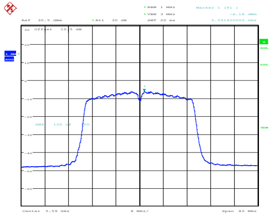
802.11ac40_5590MHz_Chain 1
