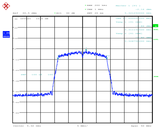
802.11ac20_5320MHz_Chain 0
