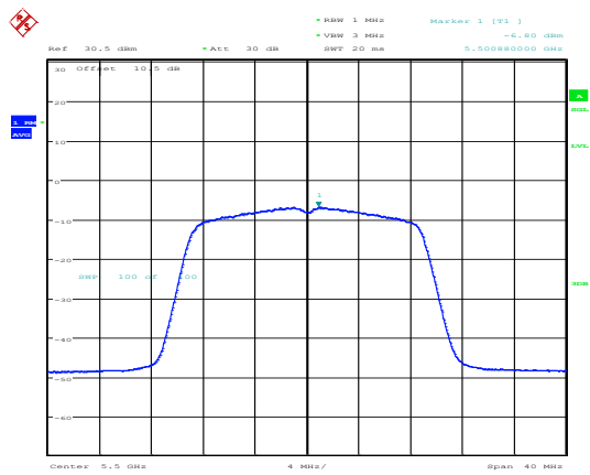
802.11ac20_5500MHz_Chain 0
