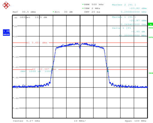
802.11ac40_5270MHz_Chain 0
