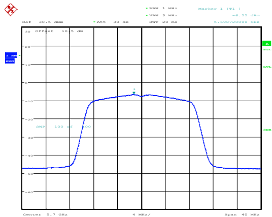
802.11n20_5700MHz_Chain 1
