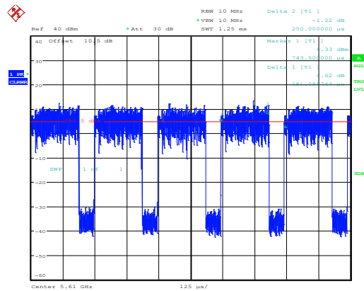
802.11ac80_5610MHz_Chain 0
