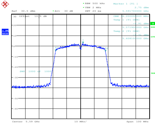
802.11ac40_5590MHz_Chain 0
