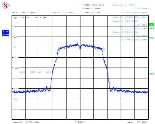
802.11a_5720MHz_Chain 0
