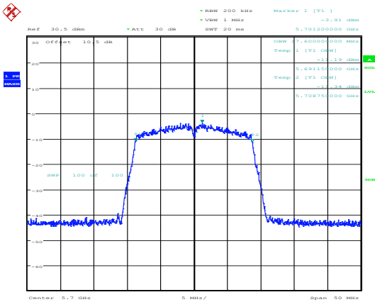
802.11ac20_5700MHz_Chain 0
