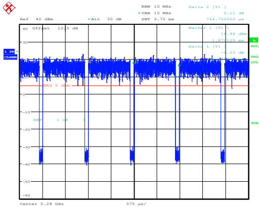
802.11ac20_5280MHz_Chain 0
