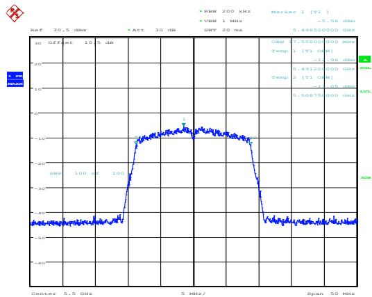
802.11ac20_5500MHz_Chain 0
