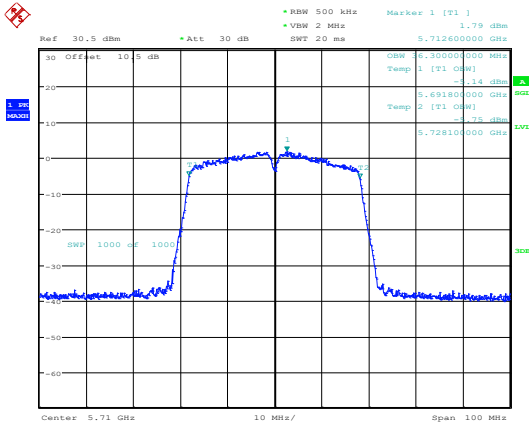
802.11ac40_5710MHz_Chain 0
