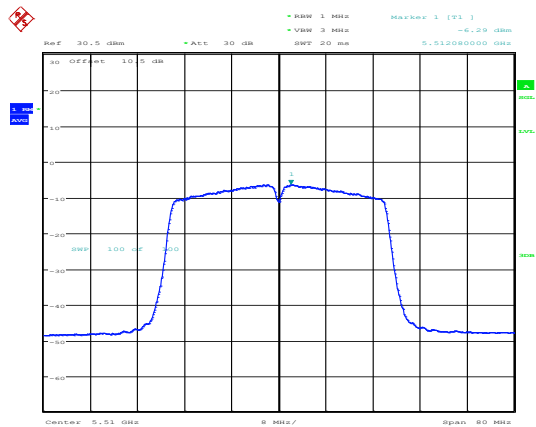
802.11n40_5510MHz_Chain 1
