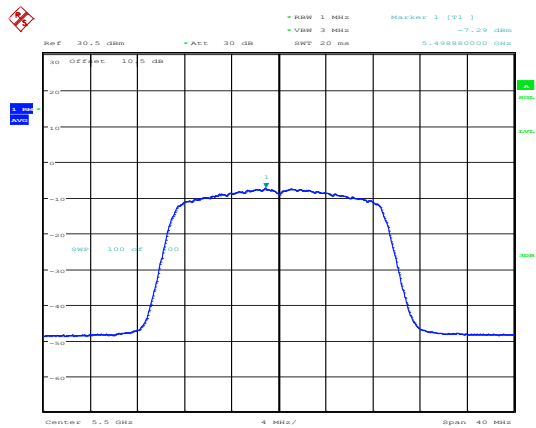
802.11ac20_5500MHz_Chain 1
