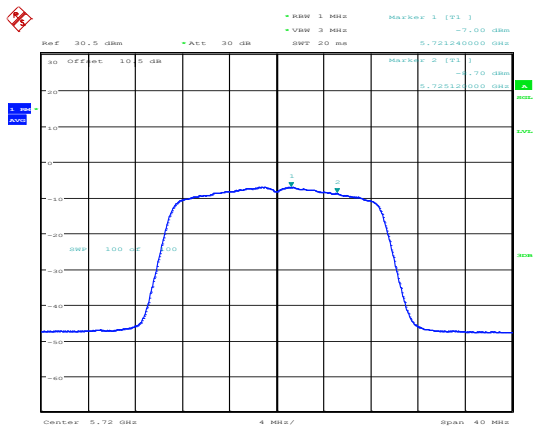
802.11n20_5720MHz_Chain 1
