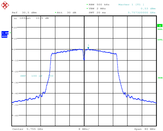
802.11ac40_5755MHz_Chain 1
