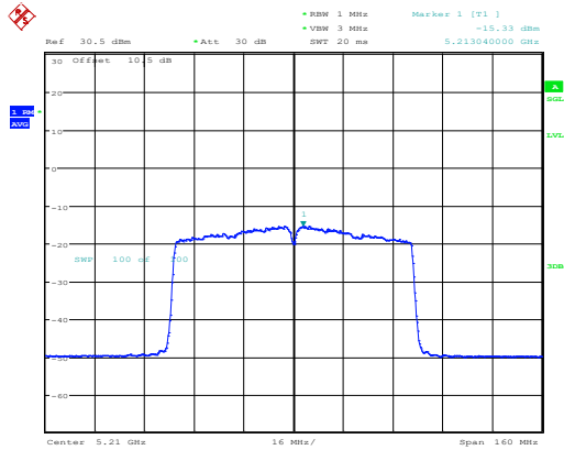
802.11ac80_5210MHz_Chain 0
