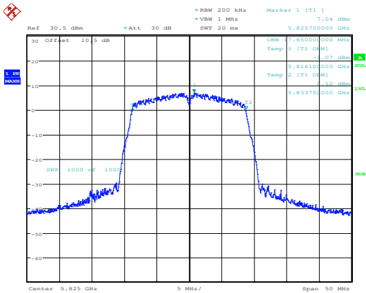
802.11ac20_5825MHz_Chain 0
