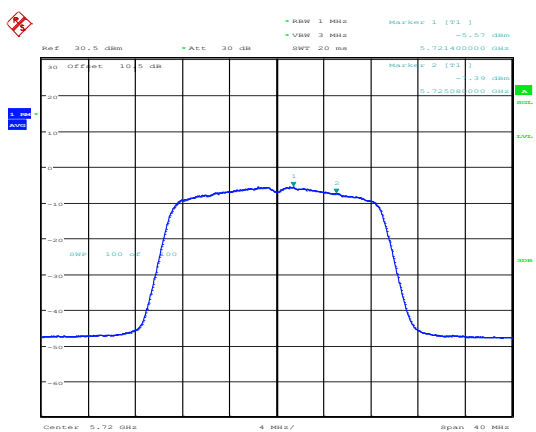
802.11ac20_5720MHz_Chain 0
