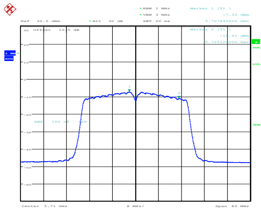
802.11ac40_5710MHz_Chain 0
