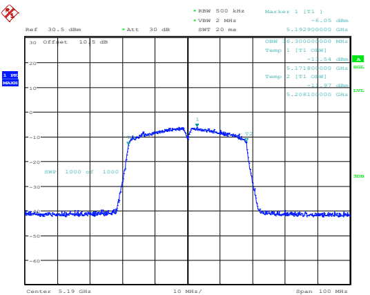
802.11ac40_5190MHz_Chain 0
