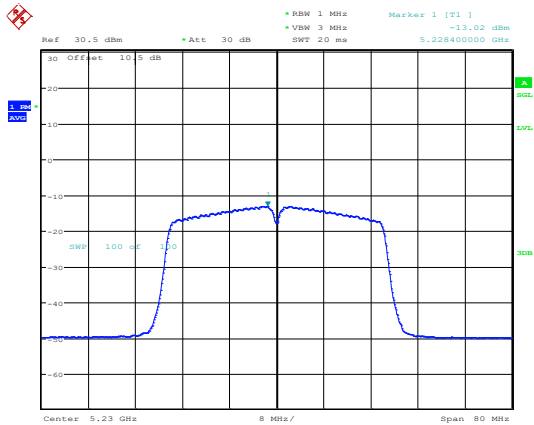
802.11n40_5230MHz_Chain 1
