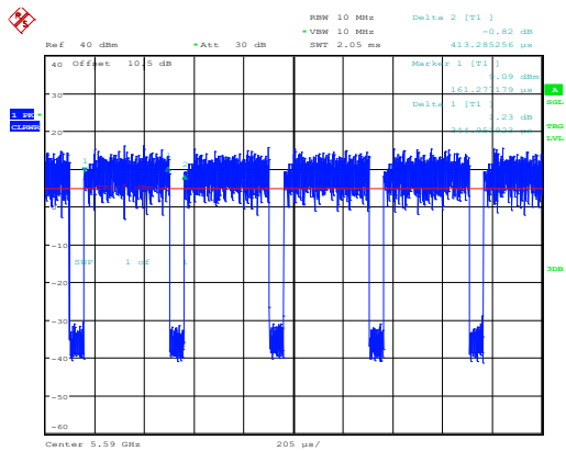
802.11ac40_5590MHz_Chain 0
