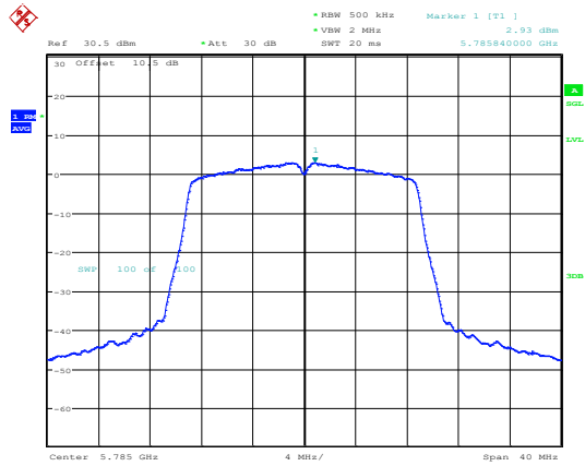
802.11ac20_5785MHz_Chain 1
