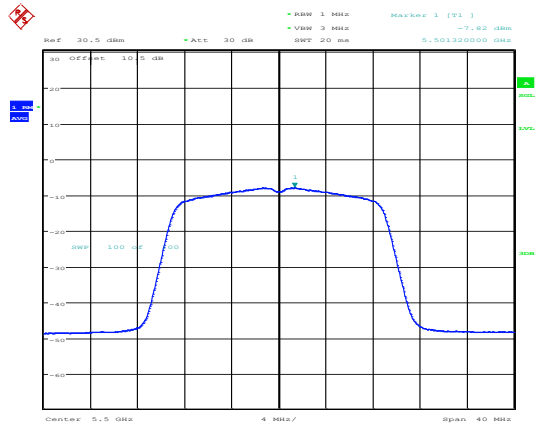
802.11n20_5500MHz_Chain 1
