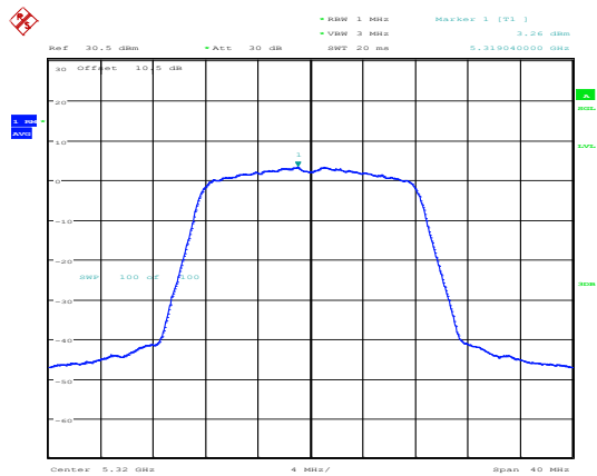
802.11a_5320MHz_Chain 0
