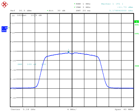
802.11ac20_5180MHz_Chain 1
