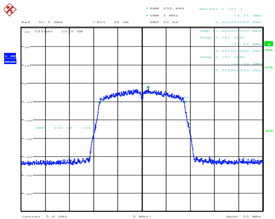
802.11ac20_5600MHz_Chain 0
