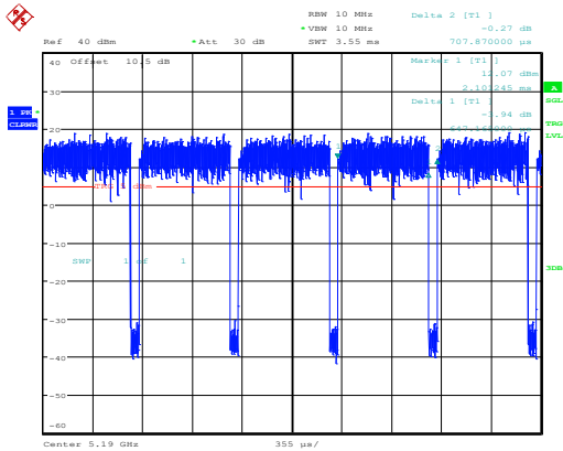
802.11n40_5190MHz_Chain 0
