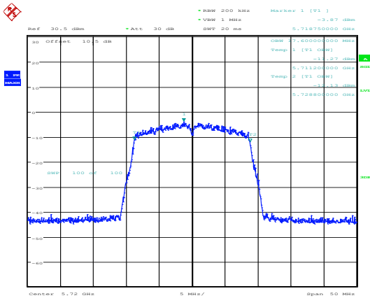
802.11ac20_5720MHz_Chain 0
