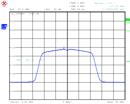
802.11ac20_5240MHz_Chain 1
