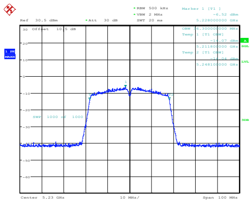
802.11ac40_5230MHz_Chain 0
