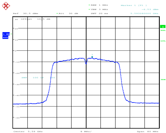
802.11ac40_5590MHz_Chain 0
