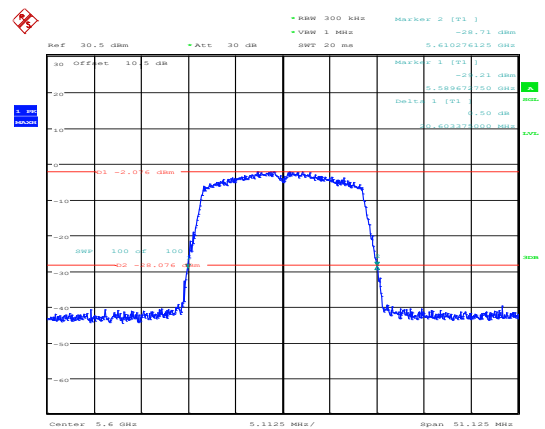
802.11ac20_5600MHz_Chain 0
