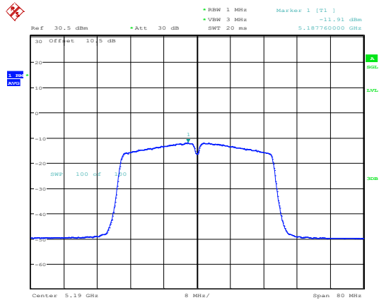
802.11n40_5190MHz_Chain 1
