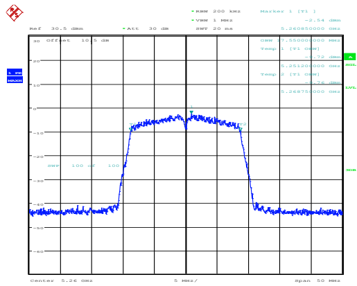
802.11n20_5260MHz_Chain 0
