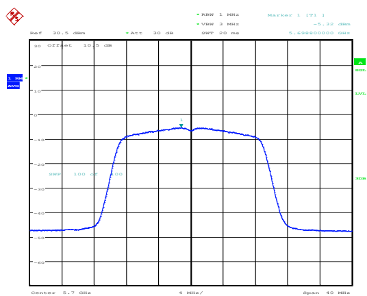
802.11ac20_5700MHz_Chain 0
