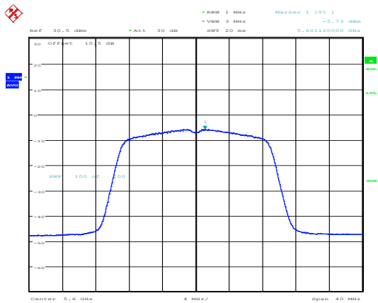
802.11ac20_5600MHz_Chain 1
