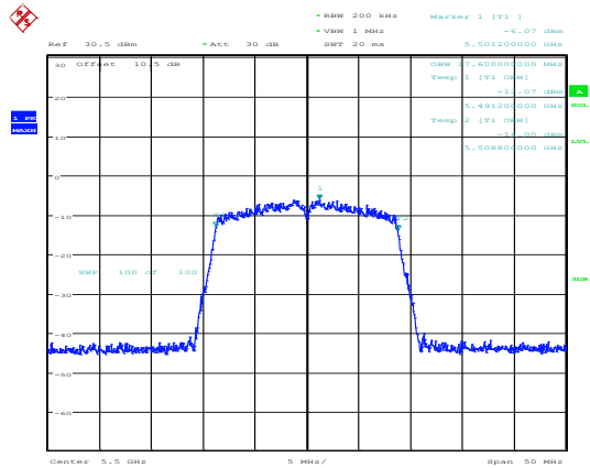
802.11n20_5500MHz_Chain 0
