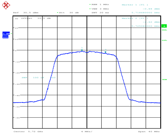
802.11a_5720MHz_Chain 1
