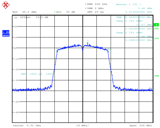
802.11n40_5310MHz_Chain 0
