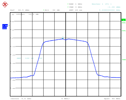
802.11a_5500MHz_Chain 1
