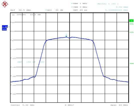
802.11a_5320MHz_Chain 1
