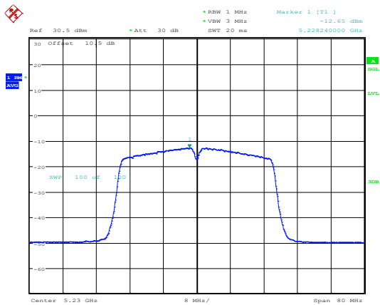
802.11n40_5230MHz_Chain 0
