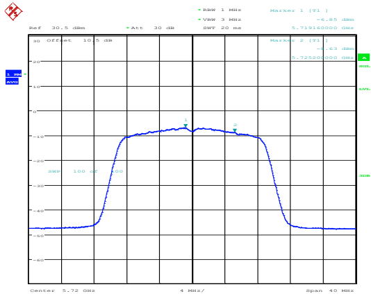
802.11ac20_5720MHz_Chain 1
