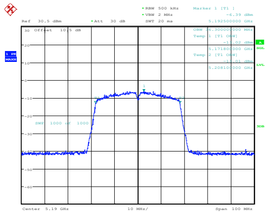
802.11n40_5190MHz_Chain 0
