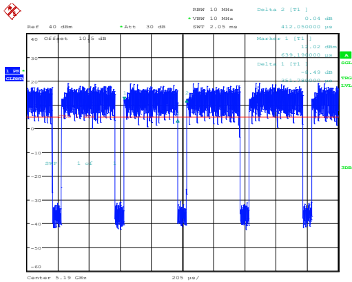
802.11ac40_5190MHz_Chain 0
