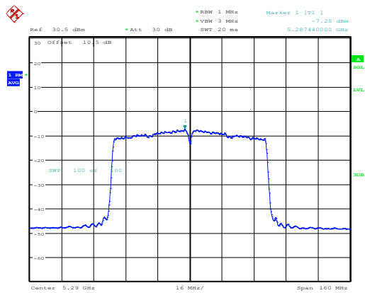
802.11ac80_5290MHz_Chain 1
