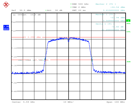
802.11n40_5590MHz_Chain 0
