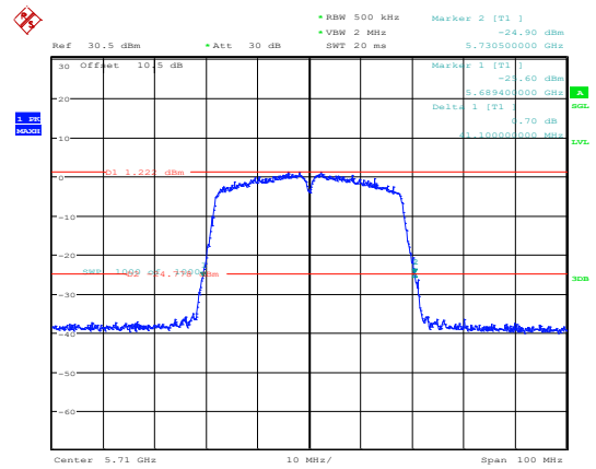
802.11n40_5710MHz_Chain 0
