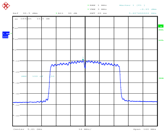
802.11ac80_5610MHz_Chain 0
