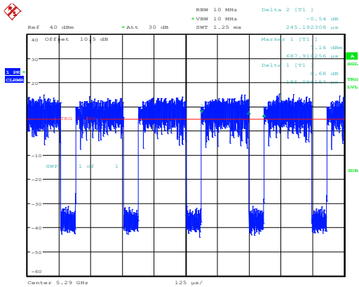
802.11ac80_5290MHz_Chain 0
