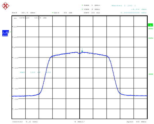
802.11ac20_5600MHz_Chain 0
