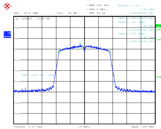
802.11ac40_5270MHz_Chain 0
