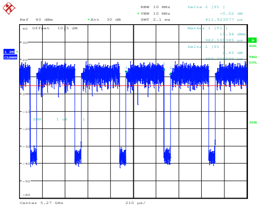
802.11ac40_5270MHz_Chain 0
