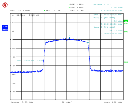
802.11ac80_5530MHz_Chain 0
