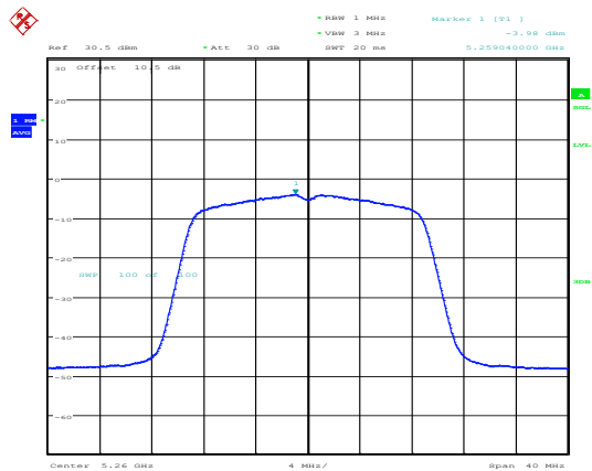
802.11n20_5260MHz_Chain 0
