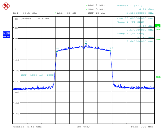
802.11ac80_5610MHz_Chain 0
