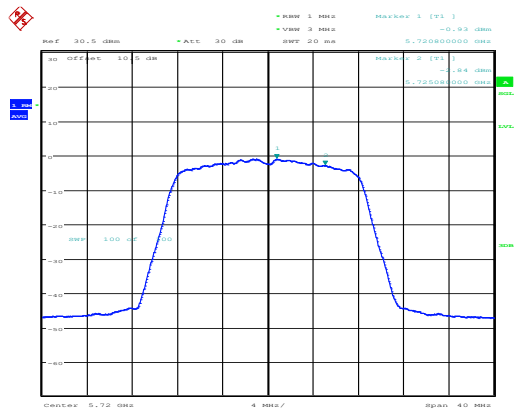
802.11a_5720MHz_Chain 0
