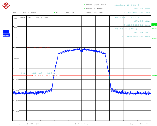
802.11ac20_5320MHz_Chain 0
