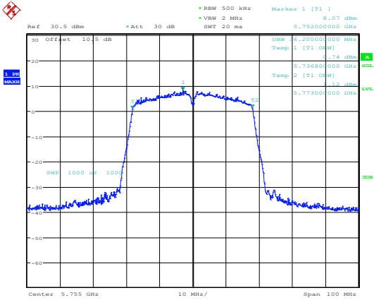
802.11ac40_5755MHz_Chain 0
