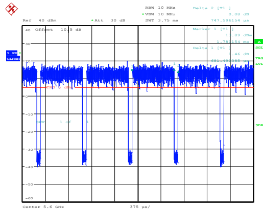
802.11ac20_5600MHz_Chain 0
