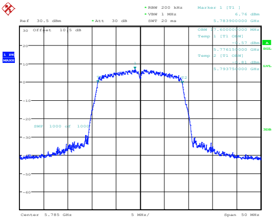
802.11ac20_5785MHz_Chain 0
