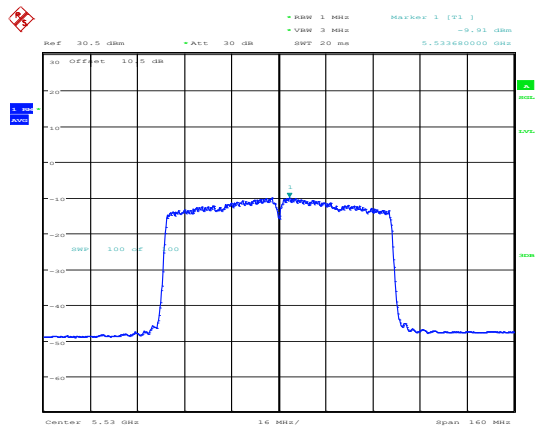
802.11ac80_5530MHz_Chain 0
