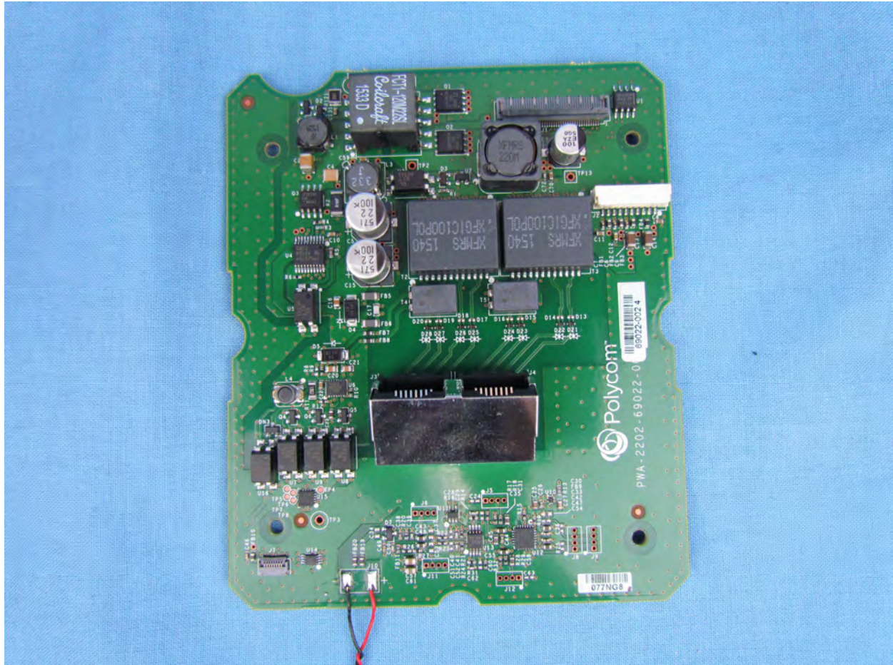
Left Arm PCB Top
