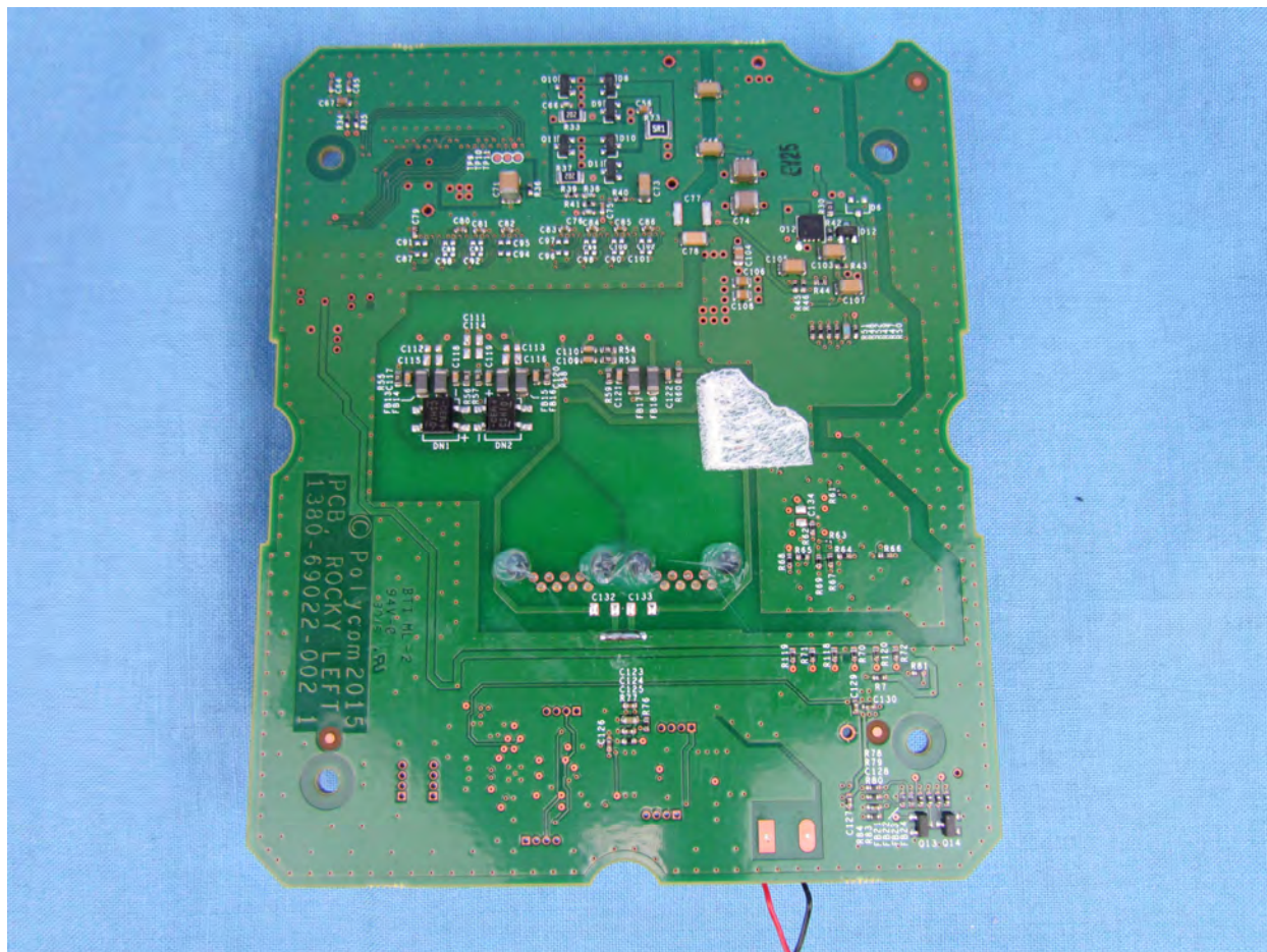
Left Arm PCB Bottom
