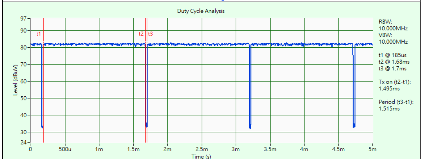
802.11ax (HE20)
