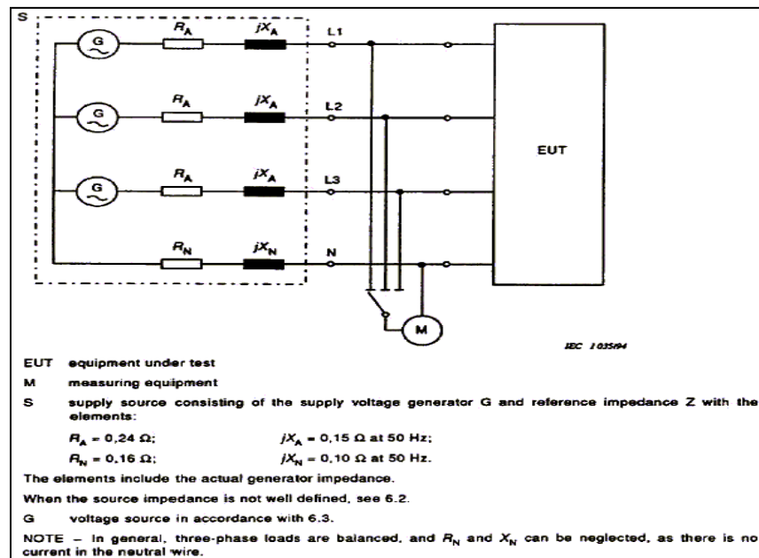
Test Circuit for EN 61000-3-3
