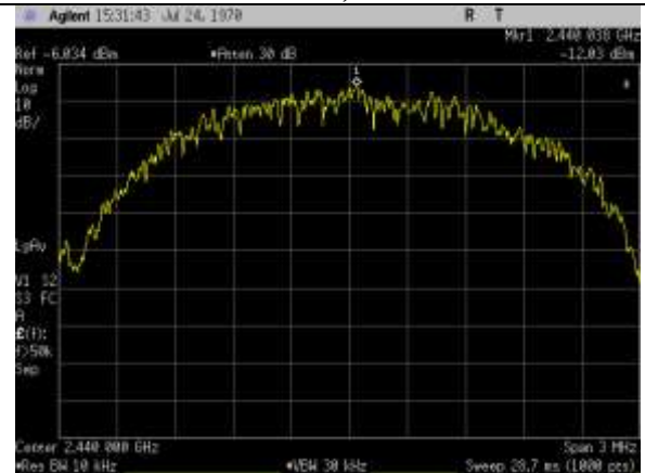
2440MHz, 2MBit
