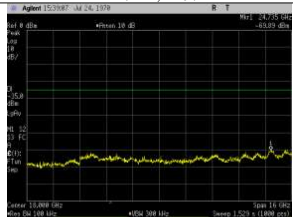
2480MHz, 2Mbit
