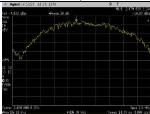
2480MHz, 1MBit
