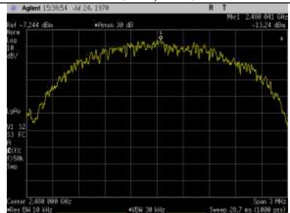
2480MHz, 2MBit
