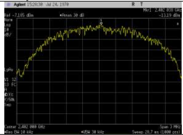
2402MHz, 2MBit
