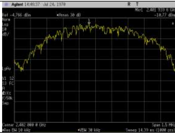
2402MHz, 1MBit
