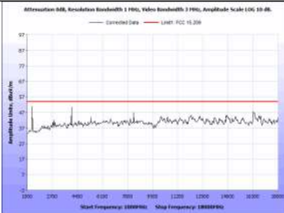
1-18GHz, Vertical
