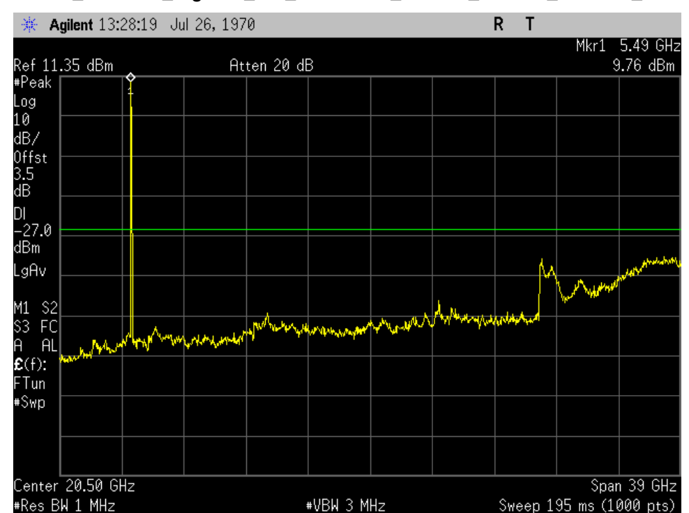
U-NII-2C_5500MHz_High Ch_100_20MHz BW_n-mode_-27dBm_1-40GHz_Port 2
