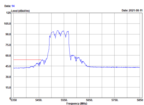
Vertical (Average)
