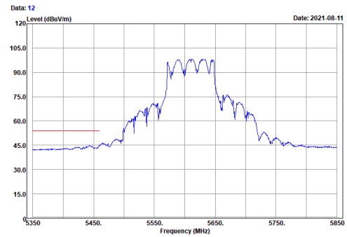
Horizontal (Average)
