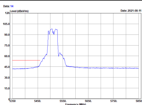
Vertical (Average)
