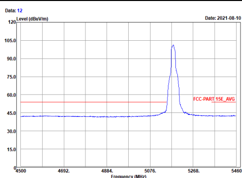
Vertical (Average)
