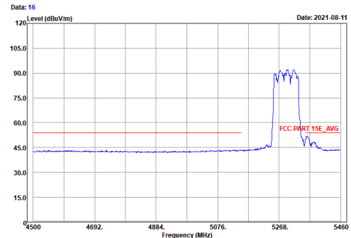
Vertical (Average)
