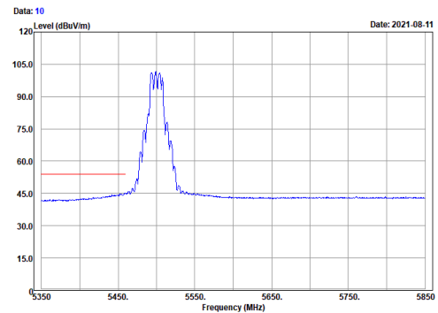
Vertical (Average)
