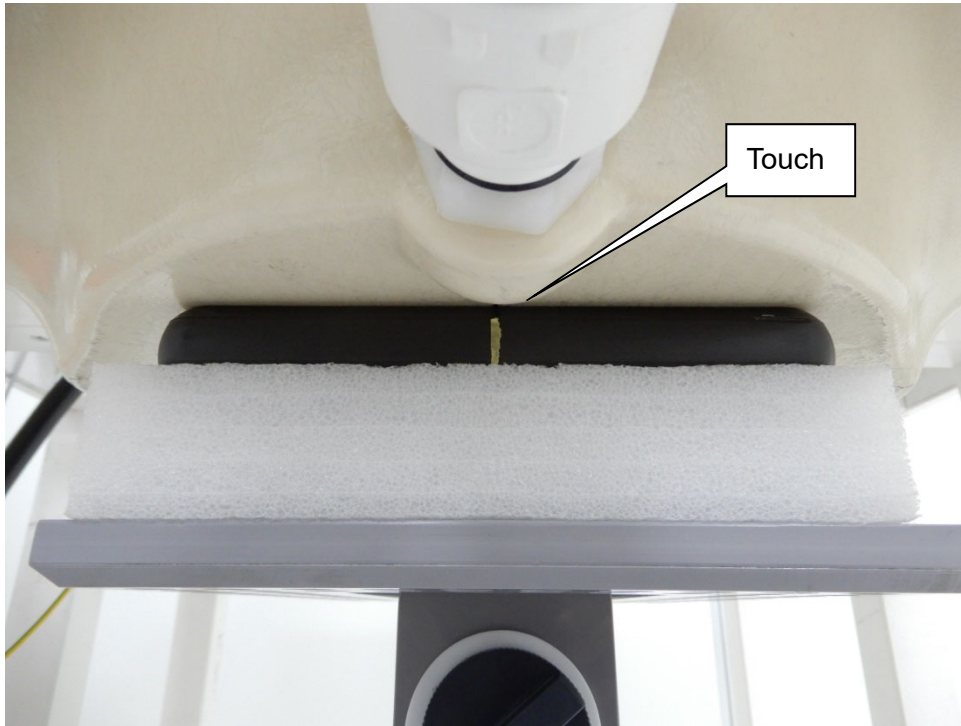
EUT Back
