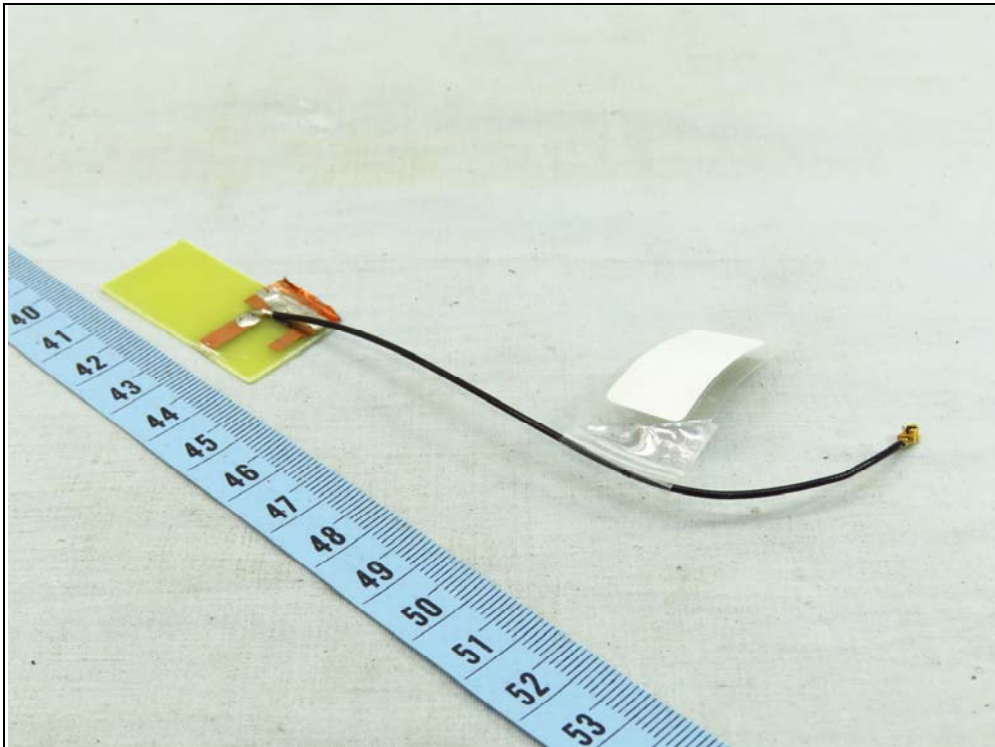
Antenna P/N: AJMQ1J-B0009
