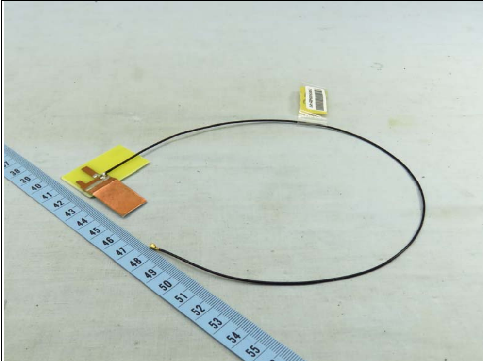
Antenna P/N: AJMQ1J-B0007
