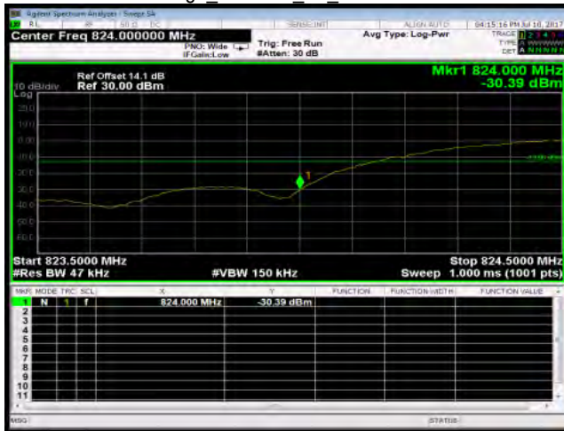
Band Edge WCDMA B5 LowCH4132-826.4
