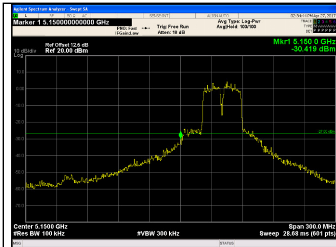
5150-5250MHz Band Edge - Low CH 5190
