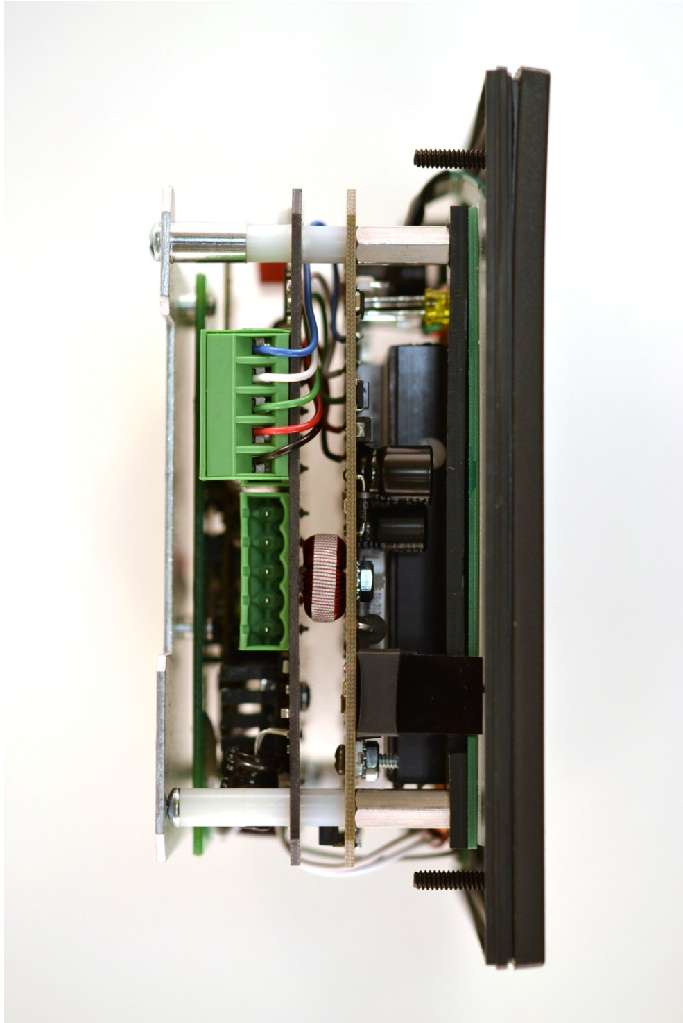
EUT Left Side
