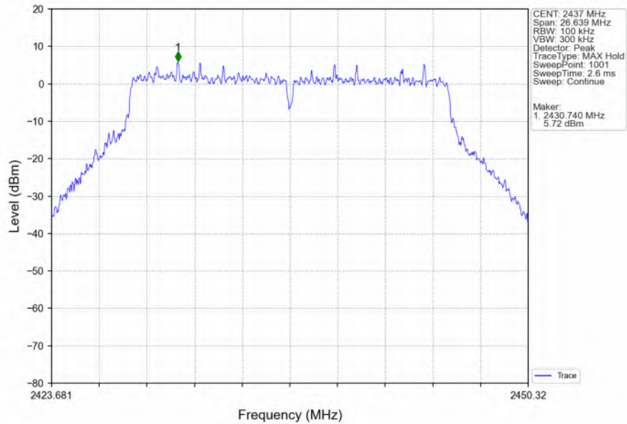
802.11n(HT20)_MCH_2437MHz_Ant2 (SISO)_NTNV
