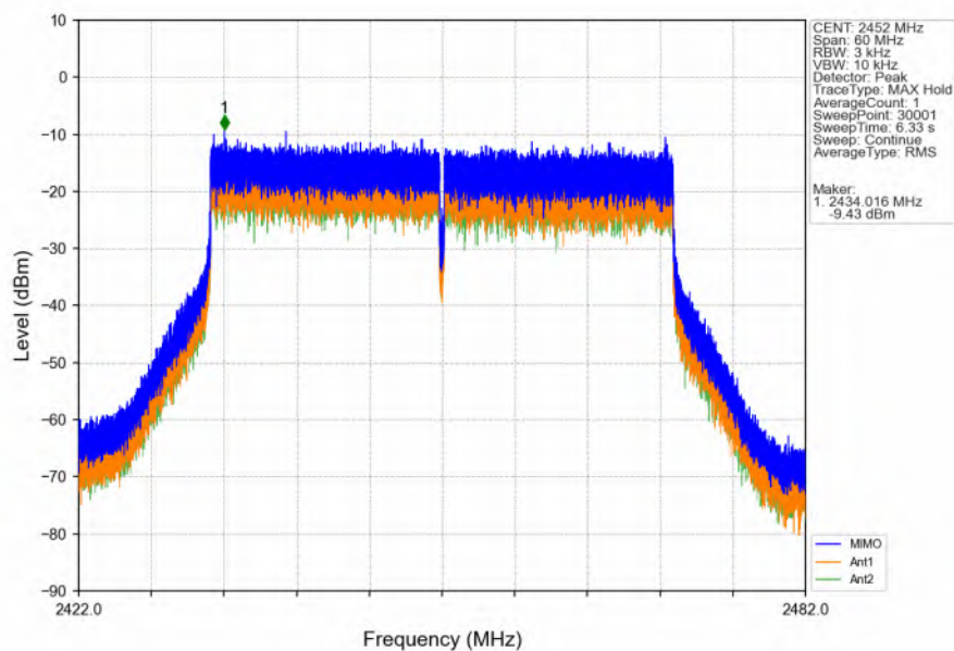
802.11be(EHT40)_HCH_2452MHz_SU_ / _MIMO_NTNV
