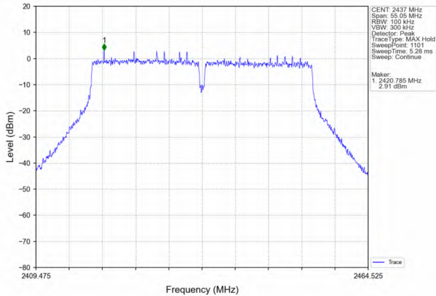
802.11n(HT40)_MCH_2437MHz_Ant2 (SISO)_NTNV
