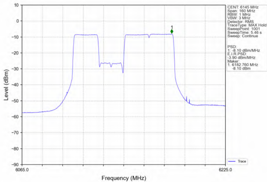
802.11be(EHT80) MCH 6145MHz 242+484 / Ant2 NTN
