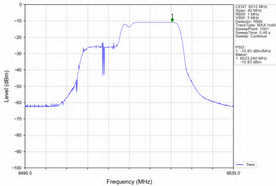
802.11be(EHT20) HCH 6515MHz 26+106 / Ant2 NTN
