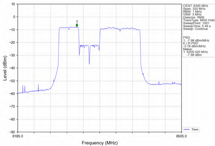
802.11be(EHT160) HCH 6345MHz 484+996 / Ant2 NTNv
