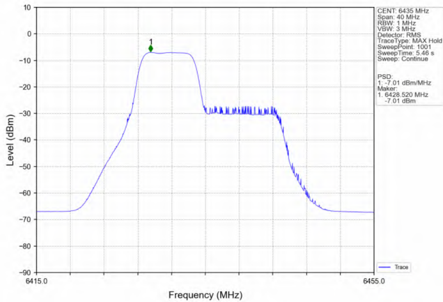
802.11be(EHT20) LCH 6435MHz 26+52 / MIMO NTN
