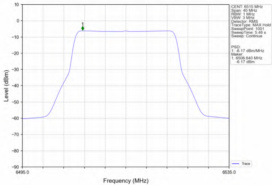
802.11be(EHT20) HCH 6515MHz SU / Ant2 NTN
