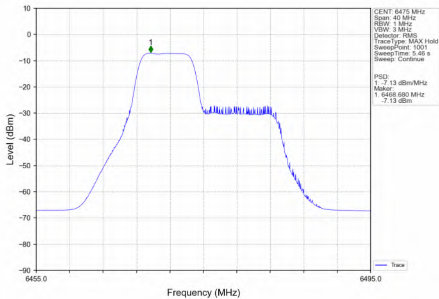
802.11be(EHT20) MCH_6475MHz_26+52 / Ant2 NTNv
