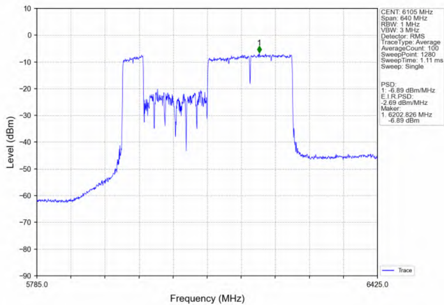
802.11be(EHT320) LCH 6105MHz P-80+40M-RU484+996+996 / Ant2 NTN
