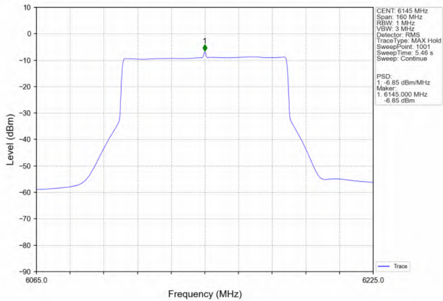
802.11be(EHT80) MCH 6145MHz SU / MIMO NTN
