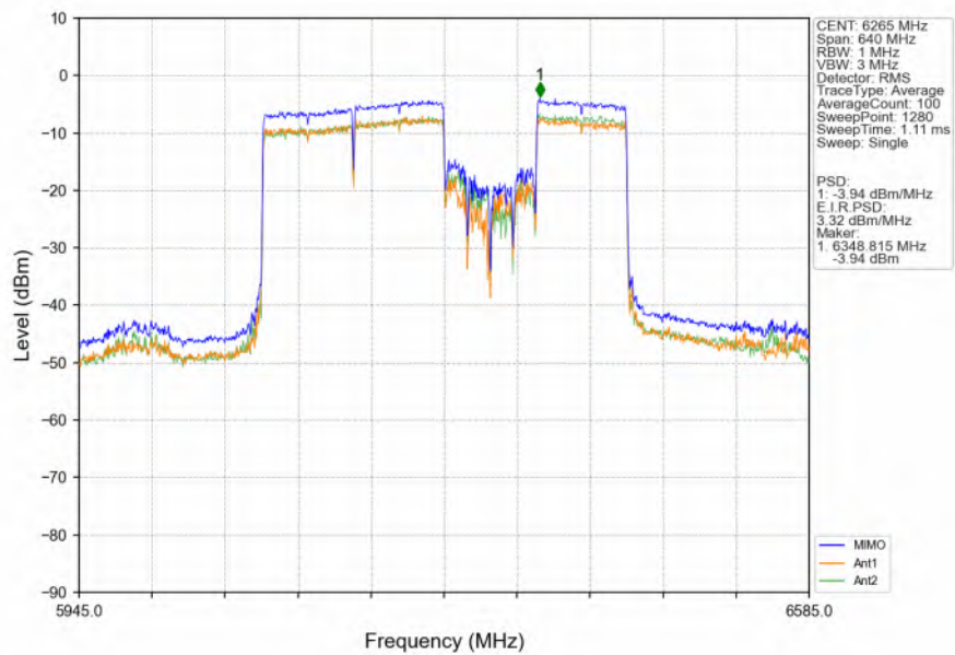
802.11be(EHT320) HCH 6265MHz 996+2X996 / MIMO NTN
