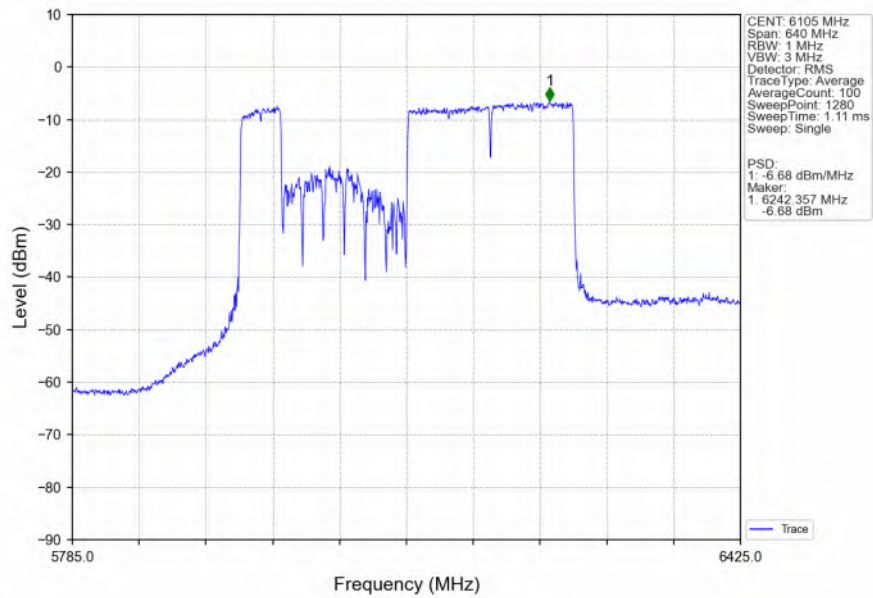
802.11be(EHT320) LCH 6105MHz 484+2X996 / Ant2 NTNv
