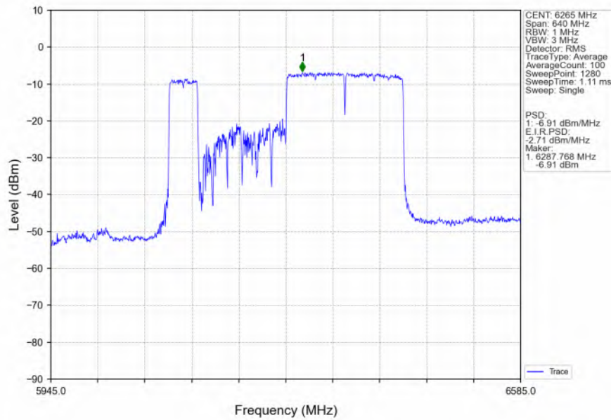
802.11be(EHT320) HCH 6265MHz P-80+40M-RU484+996+996 / MIMO NTN
