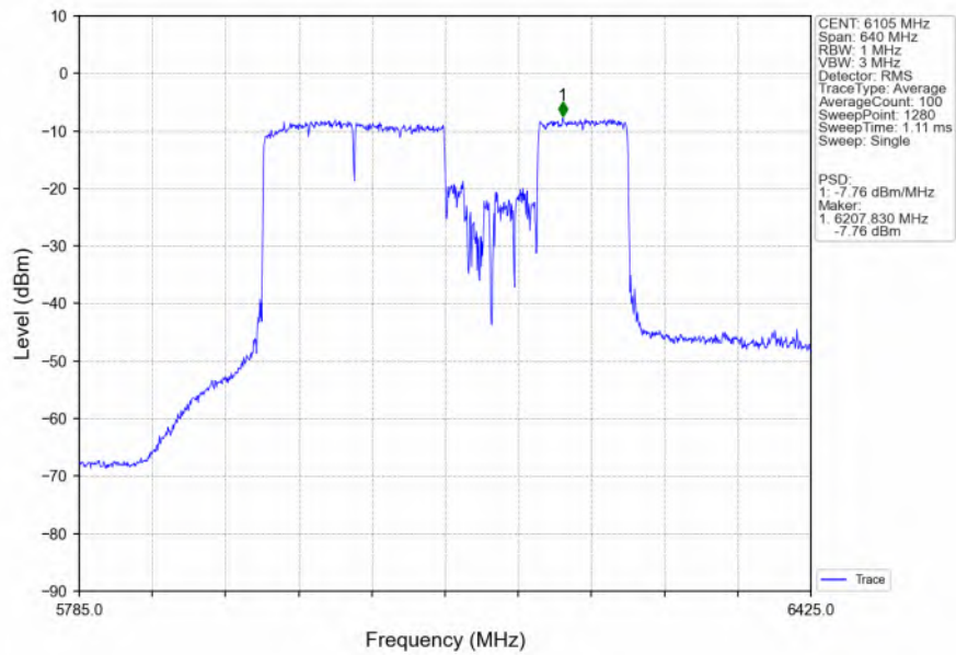
802.11be(EHT320) LCH 6105MHz P-80M-RU2X996+996 / MIMO NTN
