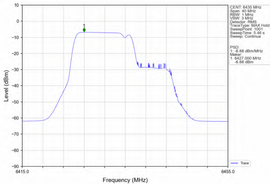
802.11be(EHT20) LCH 6435MHz 26+106 / Ant2 NTN
