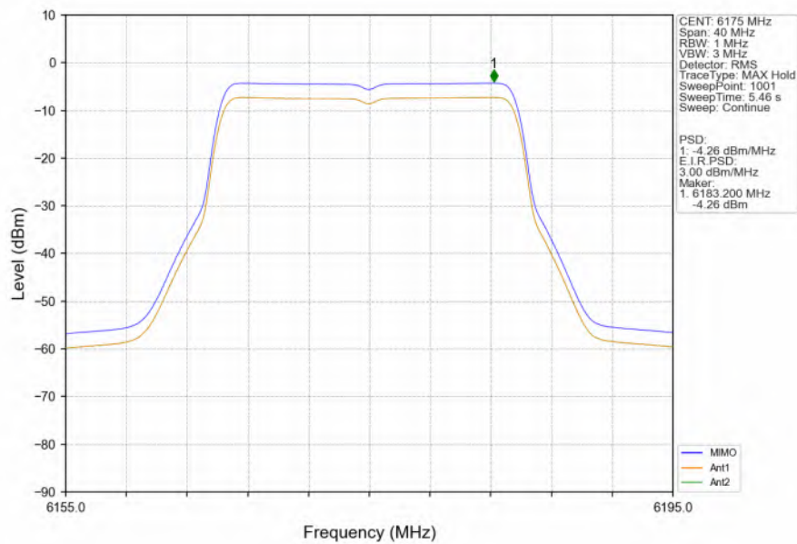
802.11be(EHT20) MCH 6175MHz SU / MIMO NTN
