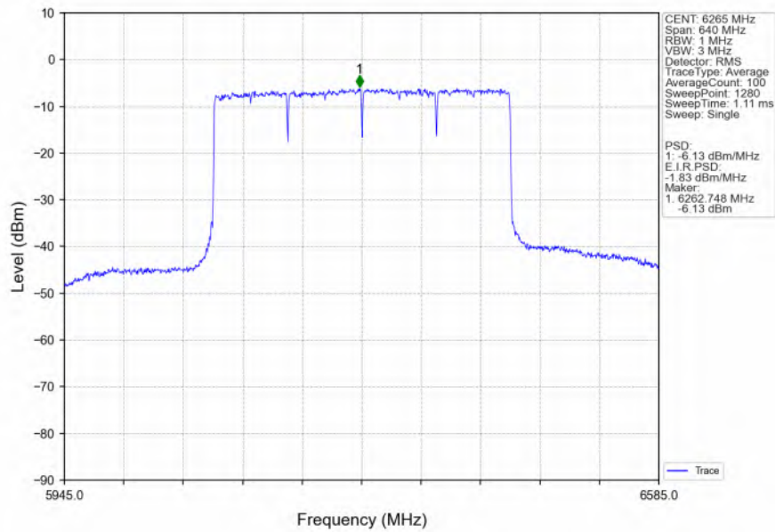
802.11be(EHT320) HCH 6265MHz SU / Ant2 NTN
