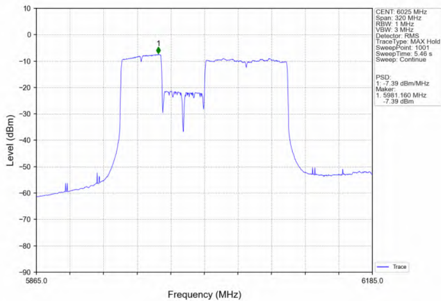
802.11be(EHT160) LCH 6025MHz 484+996 / Ant2 NTN
