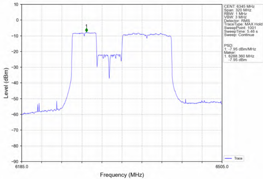
802.11be(EHT160) HCH 6345MHz 484+996 / Ant2 NTN
