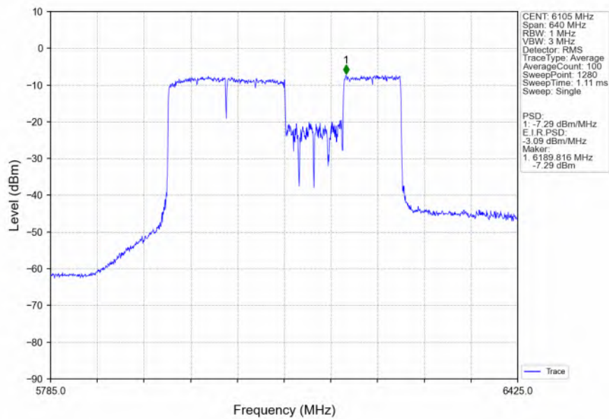
802.11be(EHT320) LCH 6105MHz 996+2X996 / Ant2 NTNv
