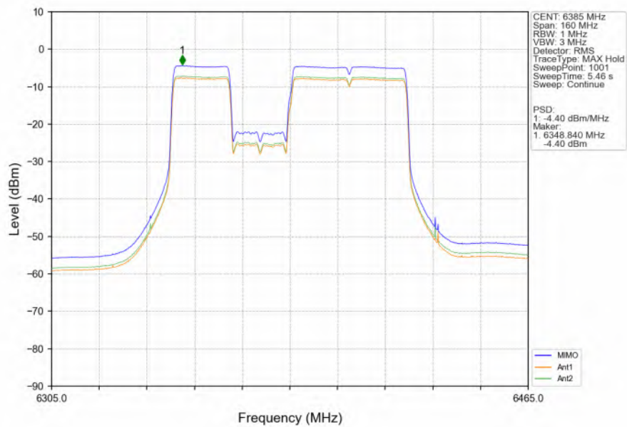
802.11be(EHT80) HCH 6385MHz 242+484 / MIMO NTN
