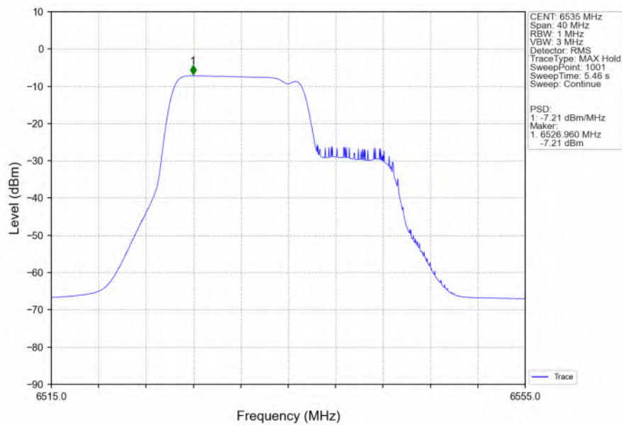
802.11be(EHT20) LCH 6535MHz 26+106 / Ant2 NTN
