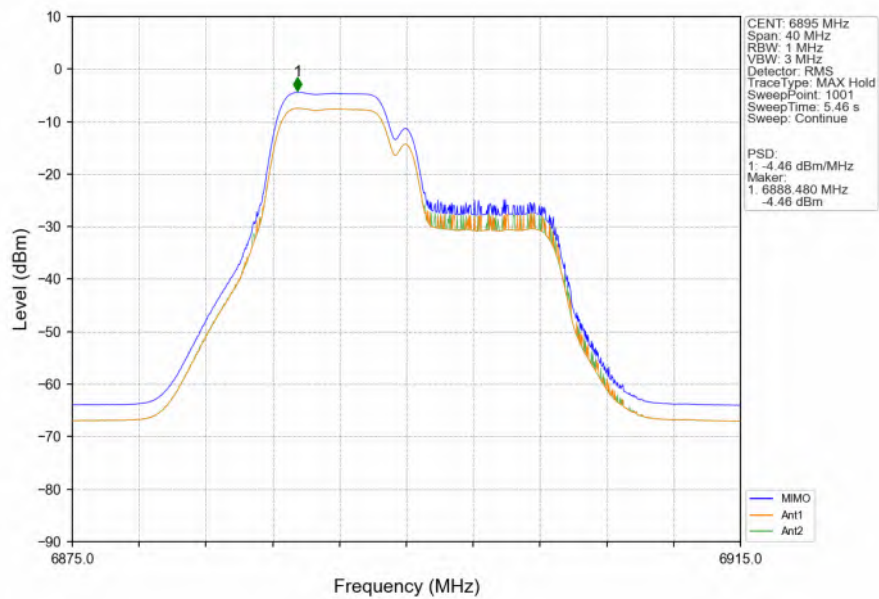
802.11be(EHT20) LCH 6895MHz 26+52 / MIMO NTN
