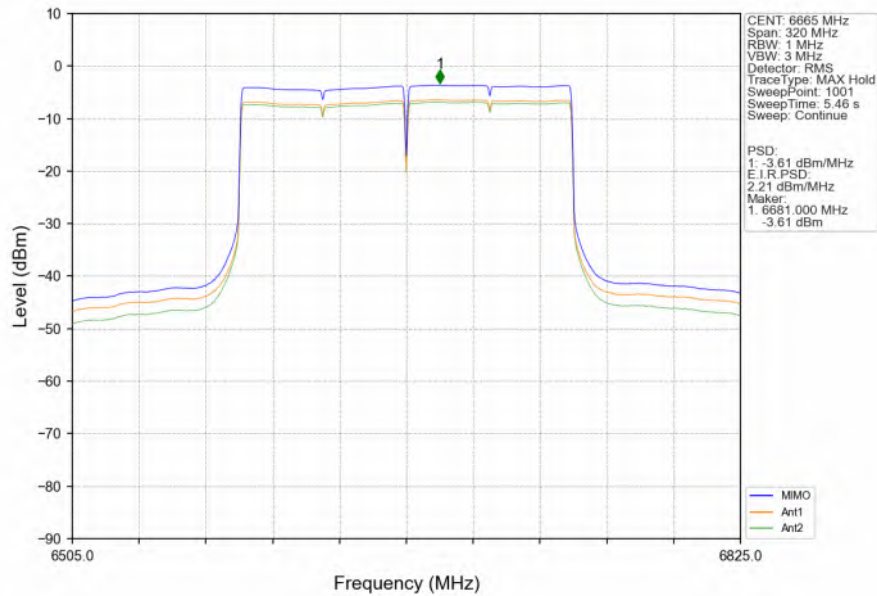
802.11be(EHT160) MCH 6665MHz SU / MIMO NTN
