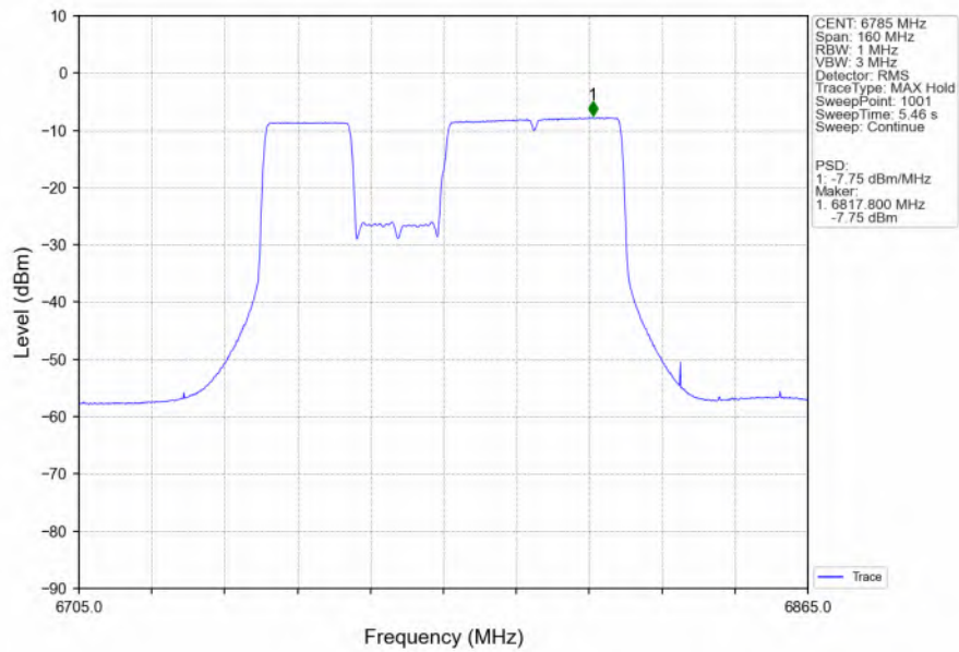
802.11be(EHT80) HCH 6785MHz 242+484 / MIMO NTN
