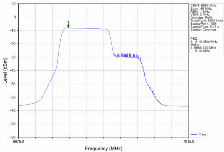
802.11be(EHT20) MCH 6995MHz 26+106 / MIMO NTN
