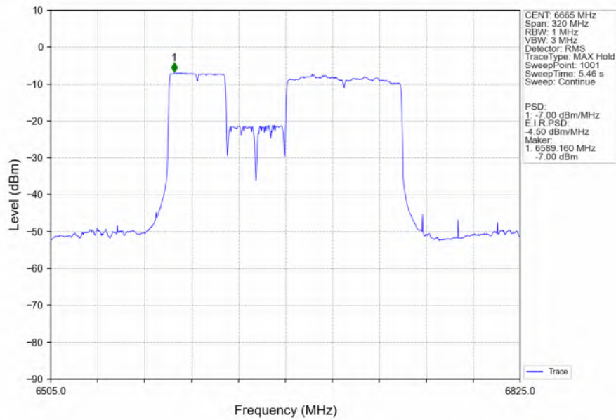
802.11be(EHT160) MCH 6665MHz 484+996 / Ant2 NTN
