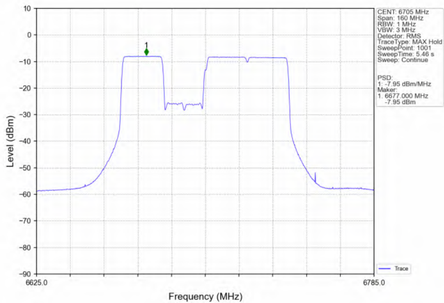
802.11be(EHT80) MCH 6705MHz 242+484 / Ant2 NTN
