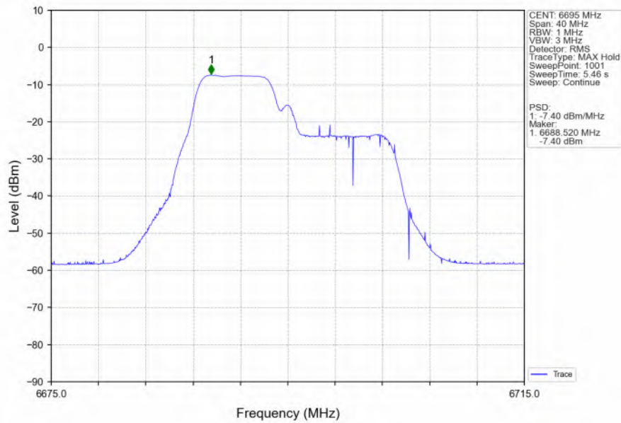
802.11be(EHT20) MCH_6695MHz_26+52 / Ant2 NTNv
