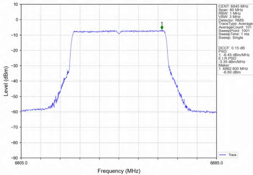
802.11be(EHT40) HCH 6845MHz SU / MIMO NTN
