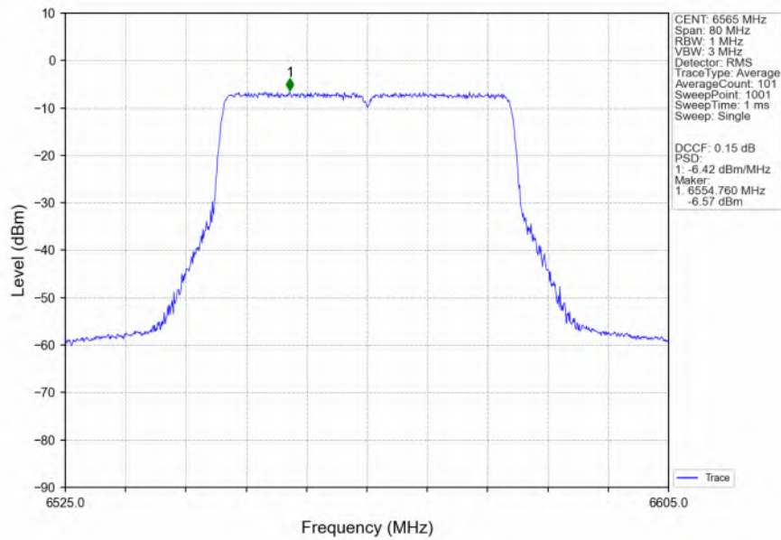
802.11be(EHT40) LCH 6565MHz SU / MIMO NTN
