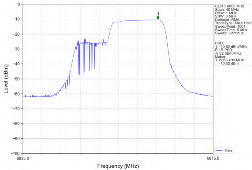
802.11be(EHT20) HCH 6855MHz 26+106 / Ant2 NTNv
