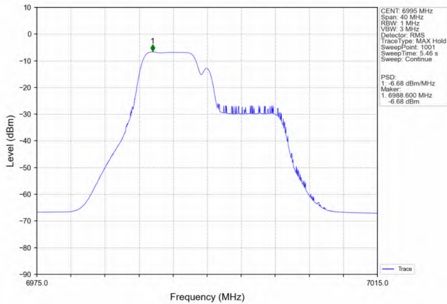
802.11be(EHT20) MCH_6995MHz_26+52 / Ant2 NTNv
