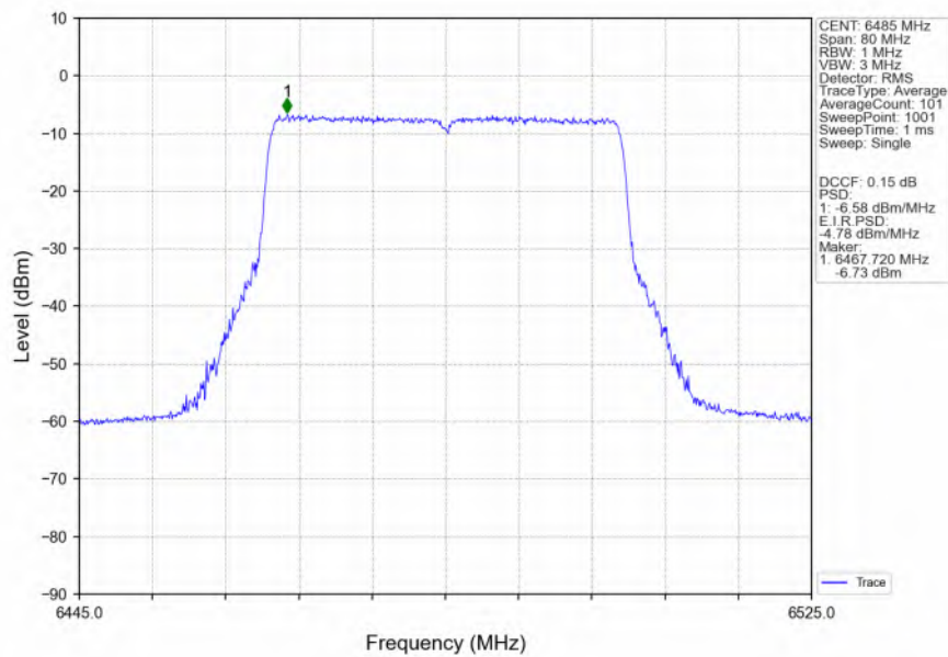
802.11be(EHT40) MCH 6485MHz SU / Ant2 NTN
