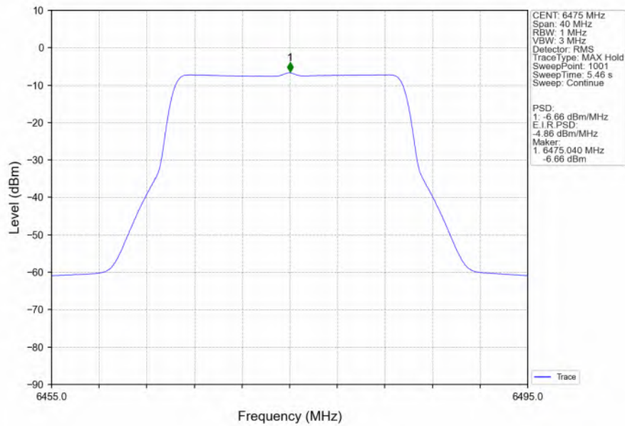
802.11be(EHT20) MCH 6475MHz SU / MIMO NTN
