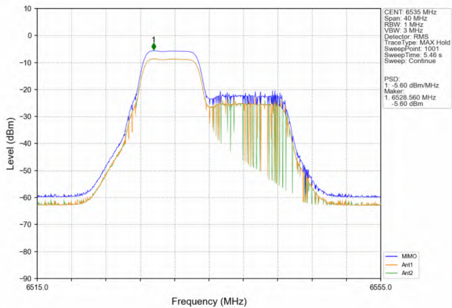
802.11be(EHT20) LCH 6535MHz 26+52 / MIMO NTN
