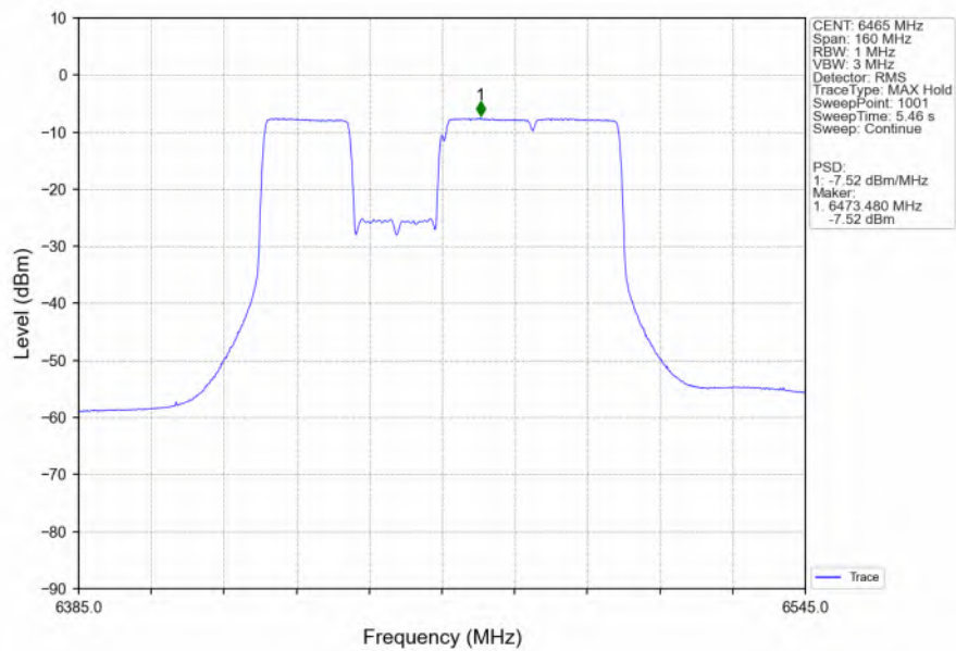
802.11be(EHT80) LCH 6465MHz 242+484 / Ant2 NTN
