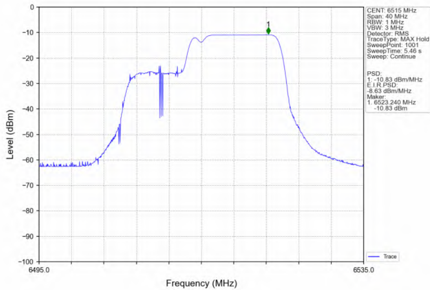
802.11be(EHT20) HCH 6515MHz 26+106 / Ant2 NTNv
