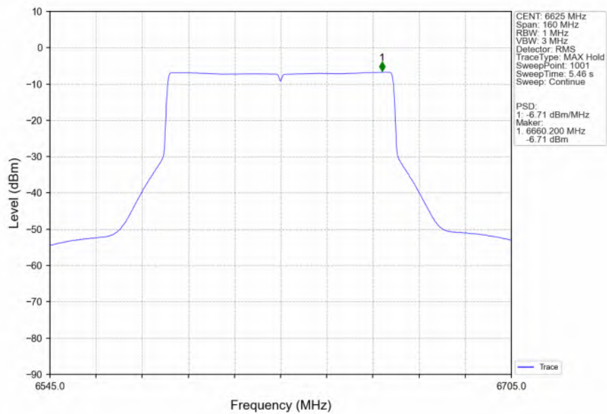
802.11be(EHT80) LCH 6625MHz SU / Ant2 NTN
