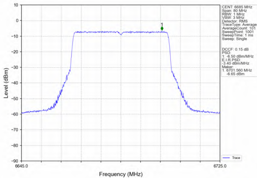
802.11be(EHT40) MCH 6685MHz SU / Ant2 NTN
