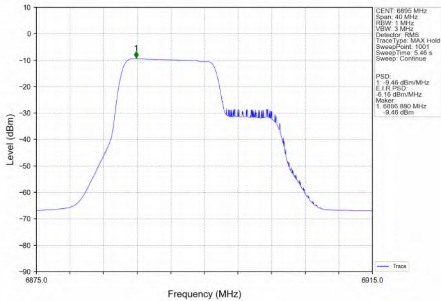
802.11be(EHT20) LCH 6895MHz 26+106 / Ant2 NTN
