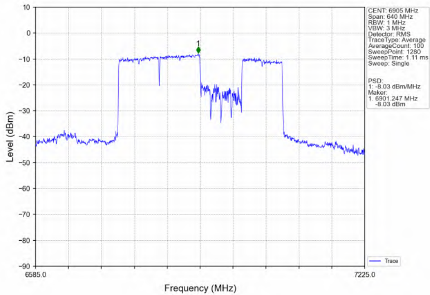
802.11be(EHT320) HCH 6905MHz P-80M-RU2X996+996 / Ant2 NTN
