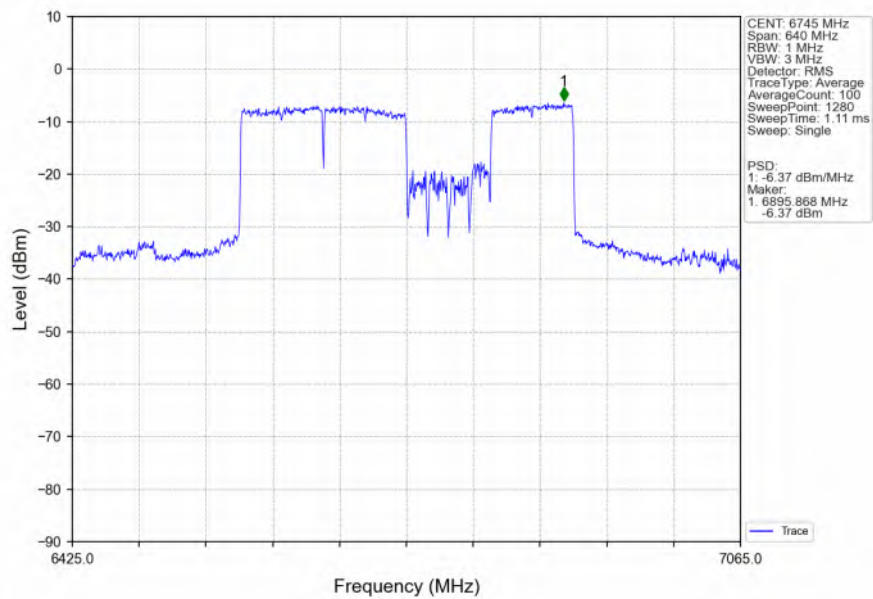
802.11be(EHT320) LCH 6745MHz 996+2X996 / Ant2 NTNv
