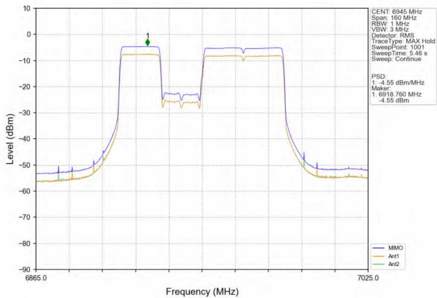
802.11be(EHT80) LCH 6945MHz 242+484 / MIMO NTN
