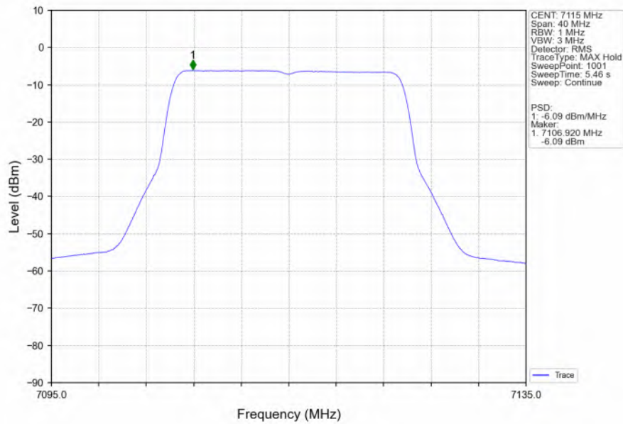
802.11be(EHT20) HCH 7115MHz SU / Ant2 NTN
