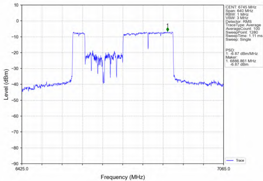
802.11be(EHT320) LCH 6745MHz P-80+40M-RU484+996+996 / Ant2 NTN
