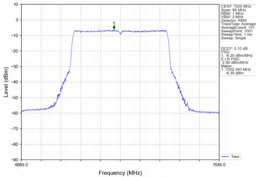
802.11be(EHT40) MCH 7005MHz SU / Ant2 NTN
