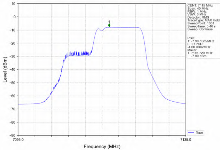
802.11be(EHT20) HCH 7115MHz 26+106 / Ant2 NTN
