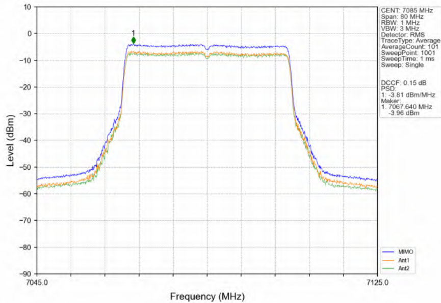
802.11be(EHT40) HCH 7085MHz SU / MIMO NTN
