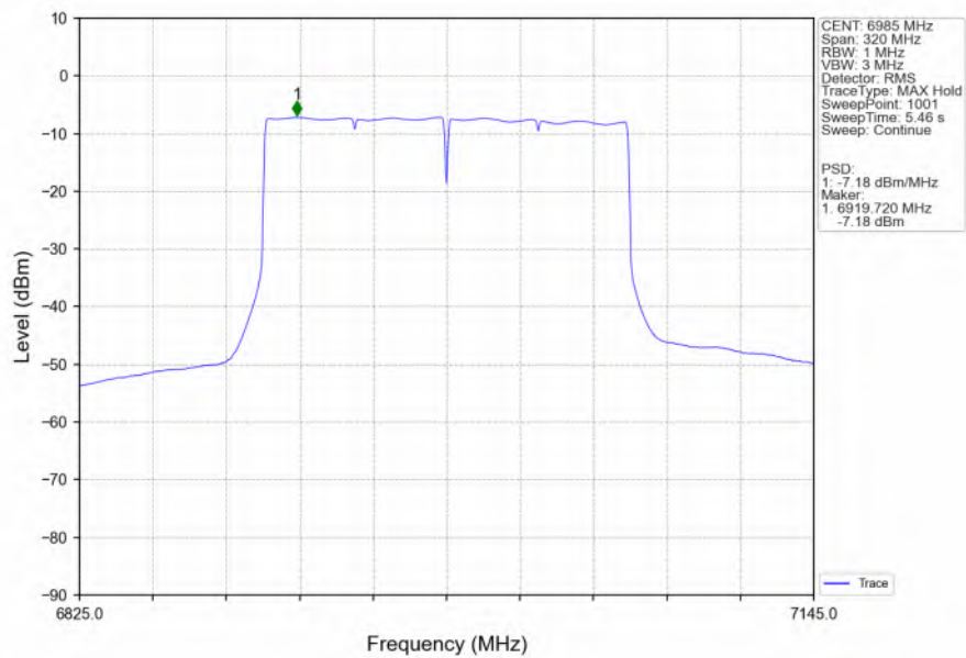
802.11be(EHT160) MCH 6985MHz SU / Ant2 NTN
