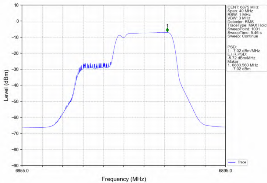
802.11be(EHT20) HCH 6875MHz 26+106 / Ant2 NTNv
