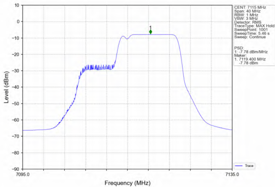
802.11be(EHT20) HCH 7115MHz 26+106 / Ant2 NTNv
