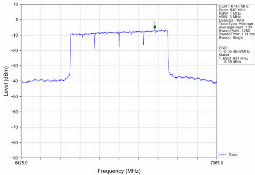
802.11be(EHT320) LCH 6745MHz SU / MIMO NTN
