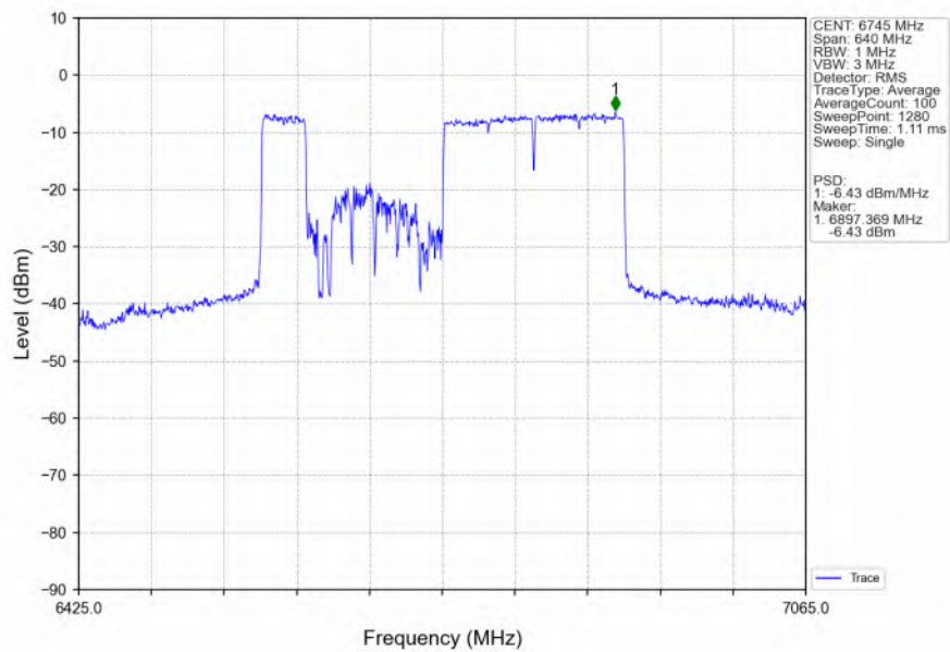
802.11be(EHT320) LCH 6745MHz 484+2X996 / Ant2 NTNv
