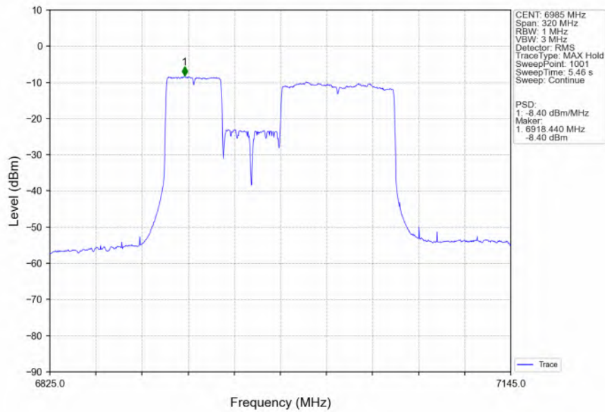
802.11be(EHT160) MCH 6985MHz 484+996 / MIMO NTN
