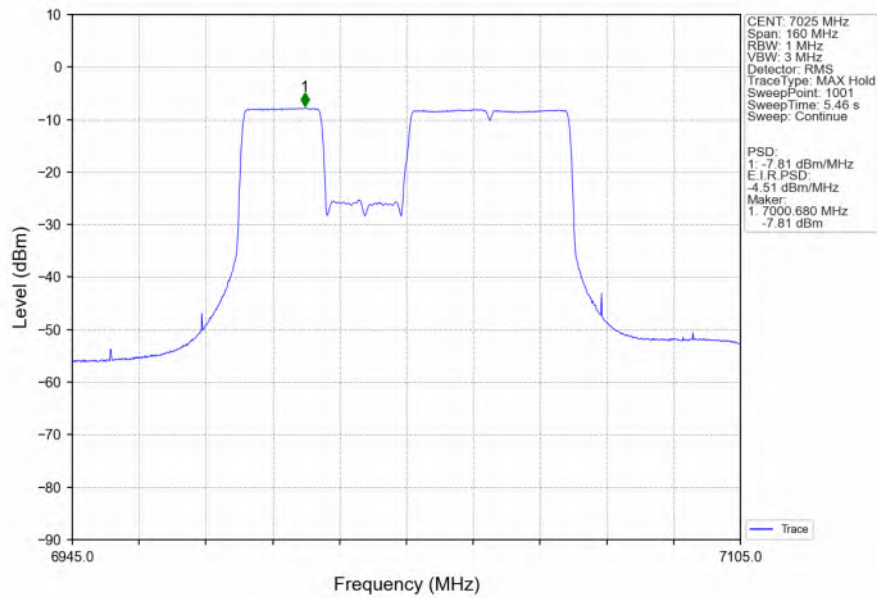
802.11be(EHT80) HCH 7025MHz 242+484 / Ant2 NTN
