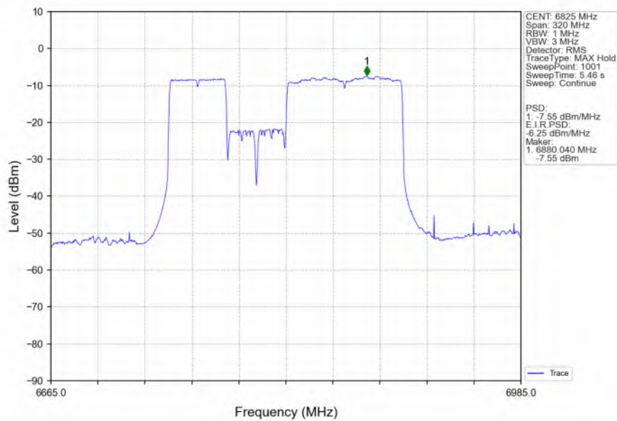
802.11be(EHT160) HCH 6825MHz 484+996 / Ant2 NTN
