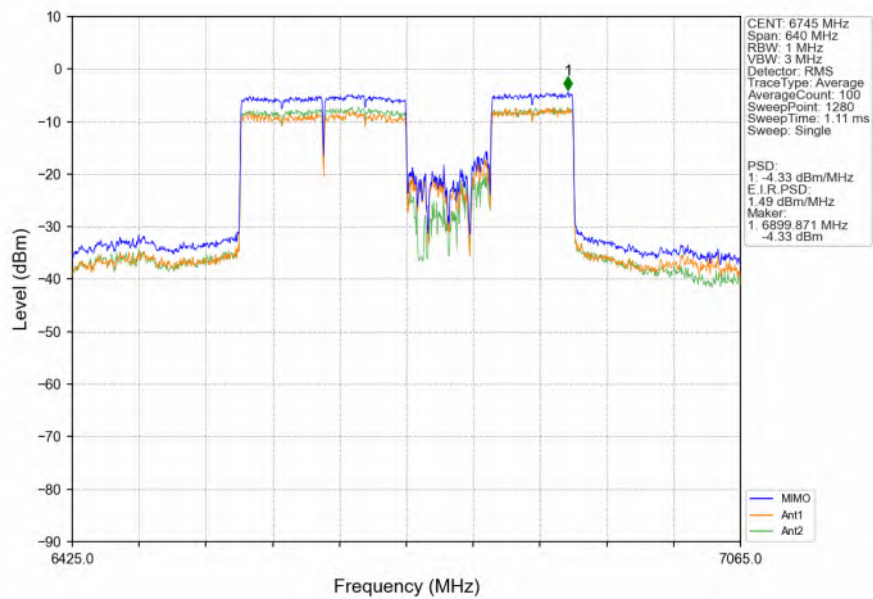
802.11be(EHT320) LCH 6745MHz P-80M-RU2X996+996 / MIMO NTN
