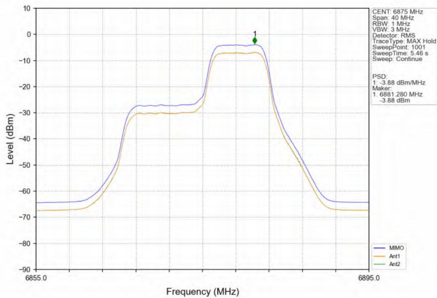
802.11be(EHT20) HCH 6875MHz 26+52 / MIMO NTN
