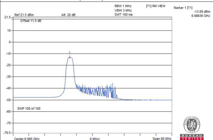
802.11ax (HE20) 26-tone RU / Chain 1 : CH 209
