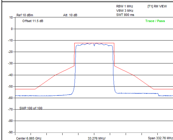
802.11ax (HE80) / Chain 0 : CH 183
