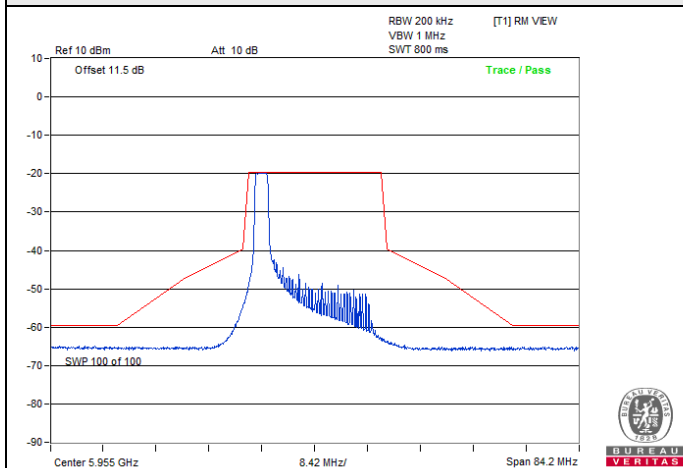
802.11ax (HE20) 26-tone RU / Chain 1 : CH 1
