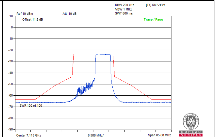
802.11ax (HE20) 106-tone RU / Chain 0 : CH 233
