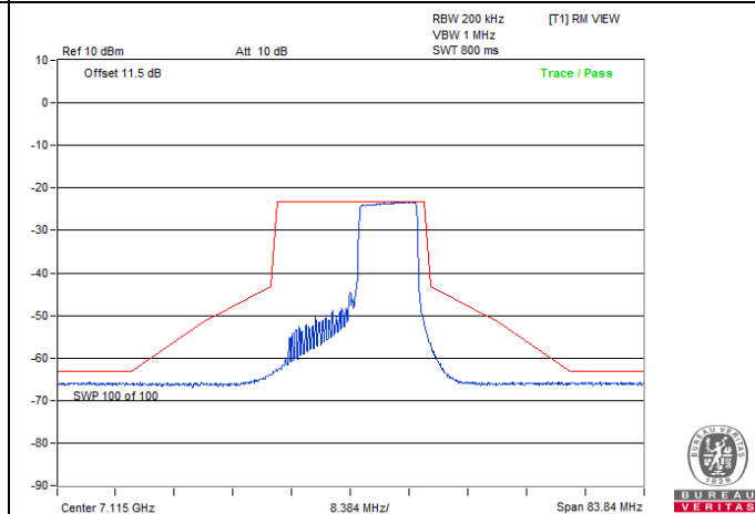
802.11ax (HE20) 106-tone RU / Chain 1 : CH 233
