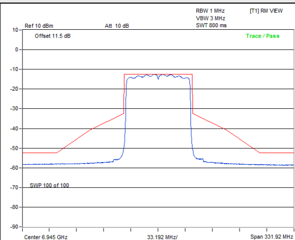
802.11ax (HE80) / Chain 0 : CH 199
