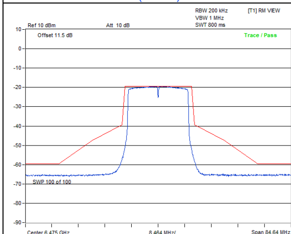
802.11ax (HE20) / Chain 1 : CH 105
