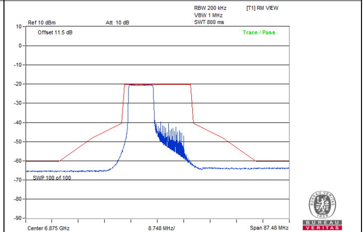
802.11ax (HE20) 106-tone RU / Chain 0 : CH 185
