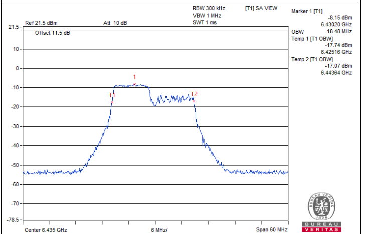
802.11ax (HE20) 106-tone RU / Chain 0 : CH 97
