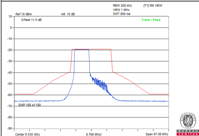
802.11ax (HE20) 106-tone RU / Chain 0 : CH 117
