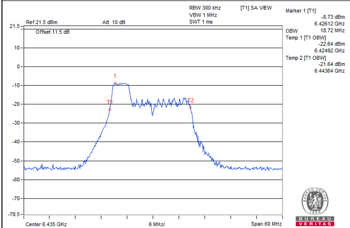
802.11ax (HE20) 52-tone RU / Chain 0 : CH 97
