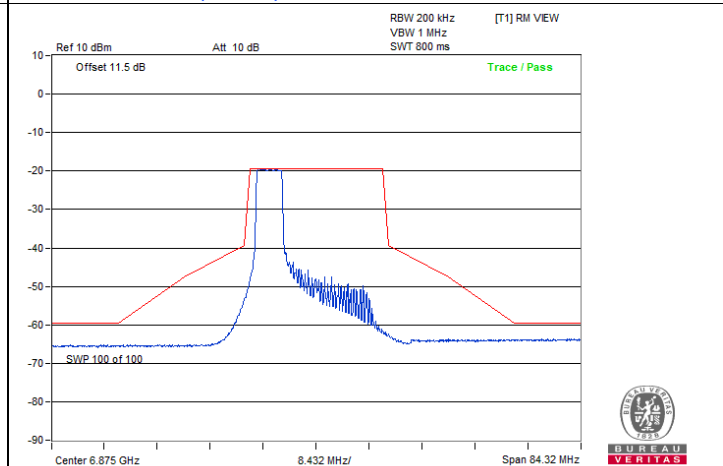
802.11ax (HE20) 52-tone RU / Chain 0 : CH 185
