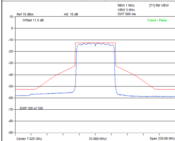
802.11ax (HE80) / Chain 0 : CH 215
