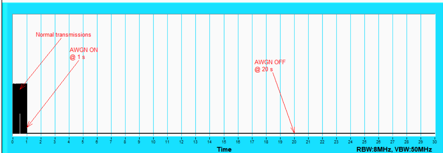
802.11ax (HE20) / CH149
