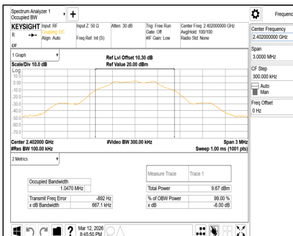
OBW_BLE 1M_LowCH00-2402MHz
