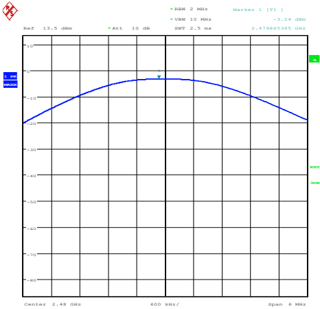
2480 MHz
