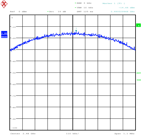
2480 MHz
