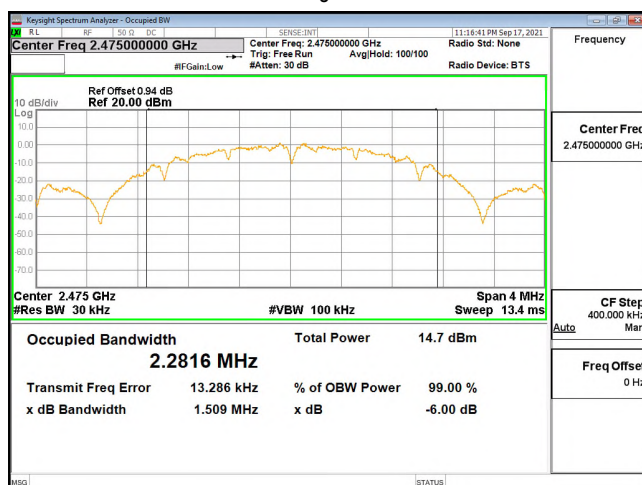
IC OBW_HighCH25-2475
