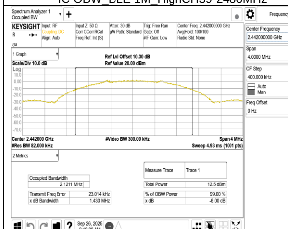
IC OBW_BLE 1M_MidCH20-2442MHz
